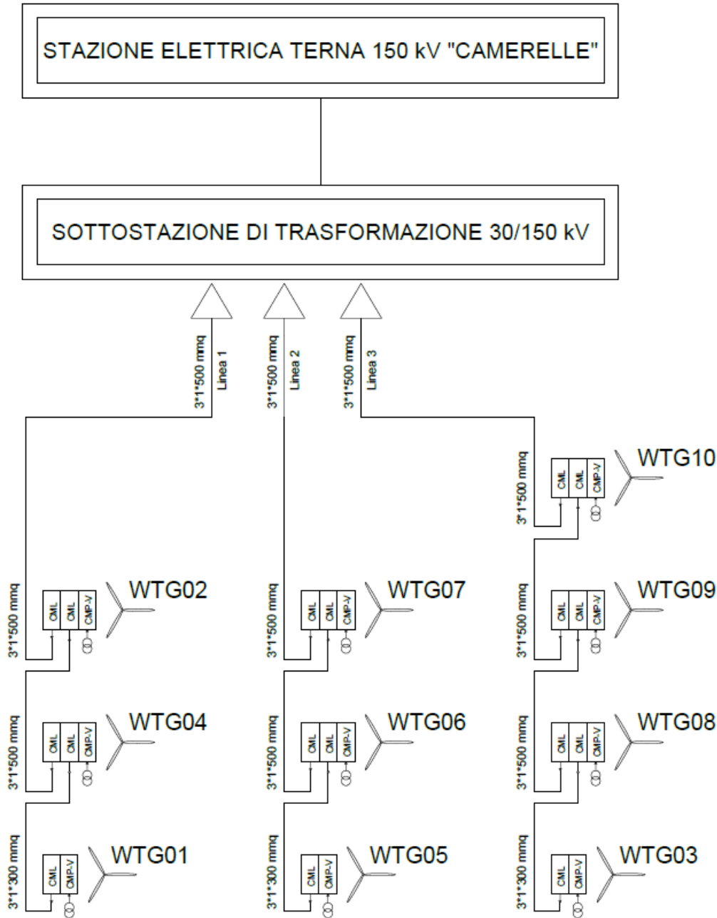
Schema Unifilare WTG
