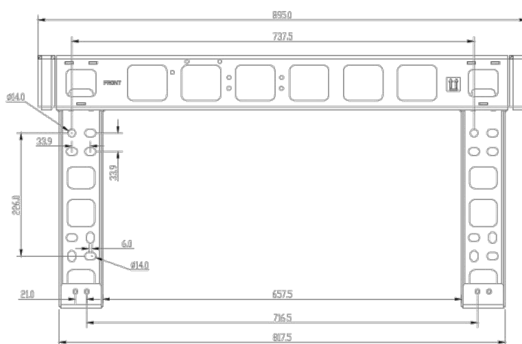
PARTICOLARE PIASTRA DI ANCORAGGIO
