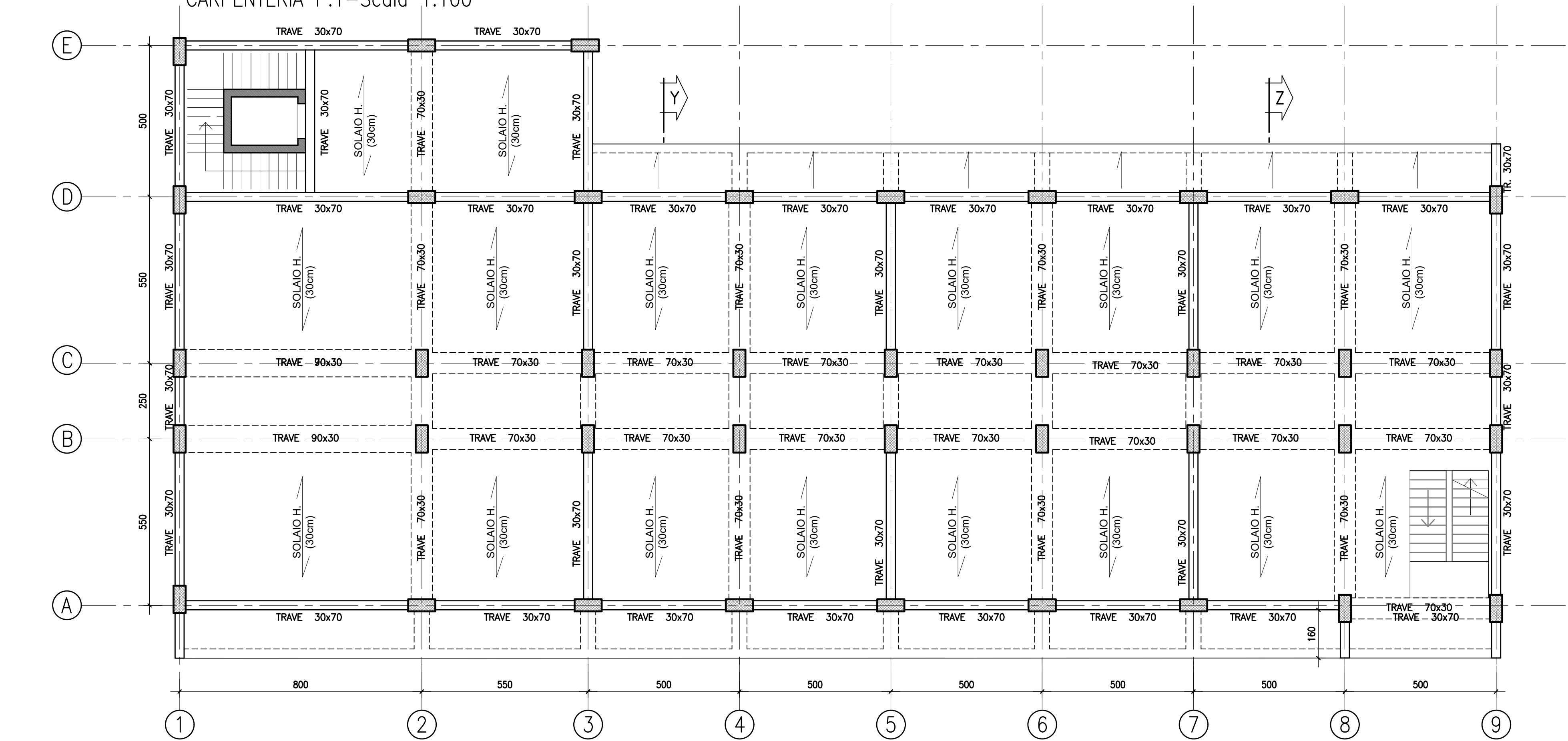
CASERMA POLIZIA STRADALE CARPENTERIA P.1–Scala 1:100
