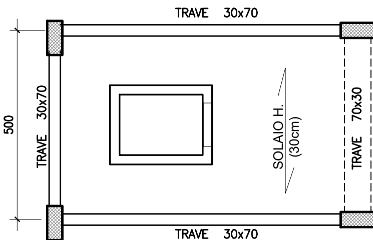
CASERMA POLIZIA STRADALE CARPENTERIA TORRINO SCALA - Scala 1:100
