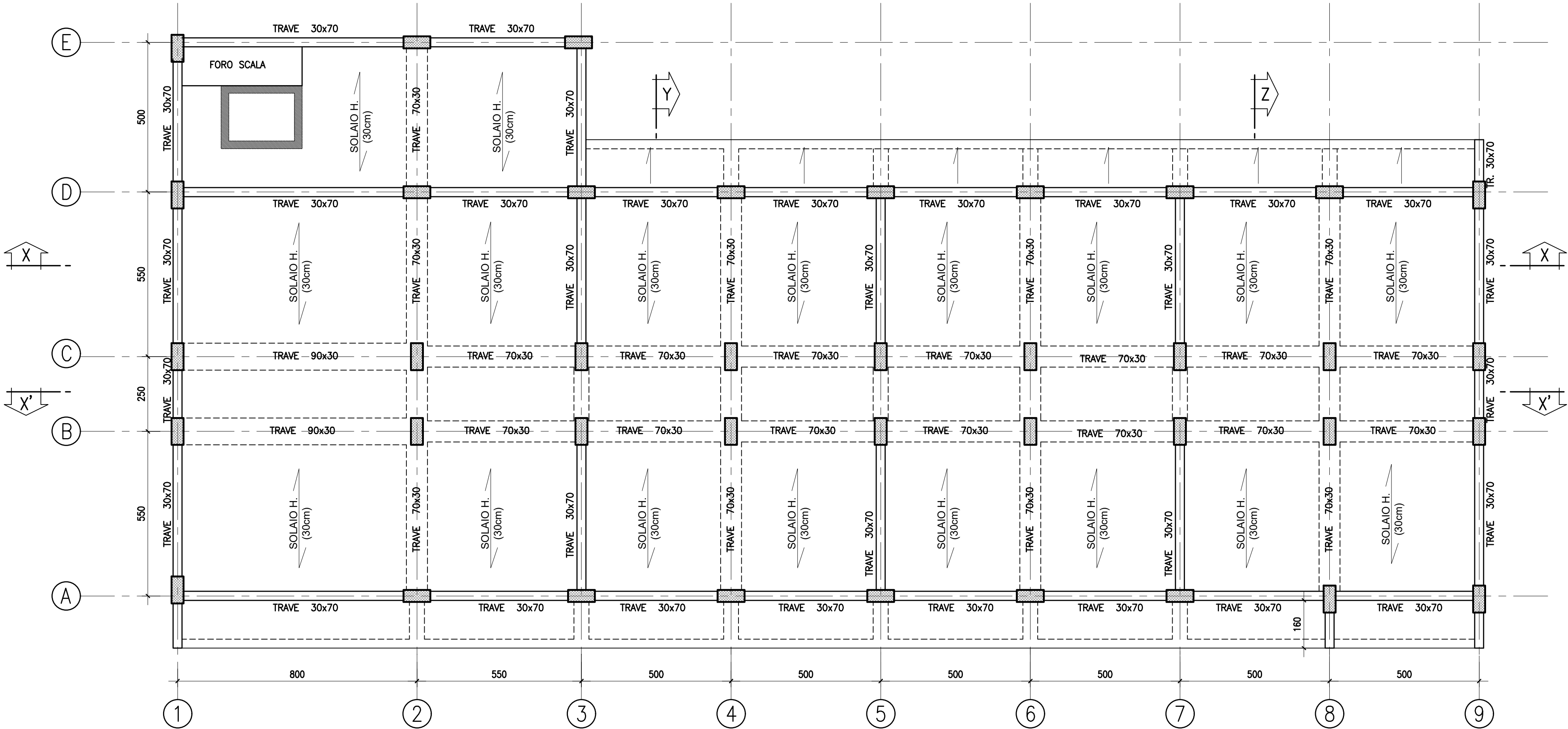
CASERMA POLIZIA STRADALE CARPENTERIA P.2 -Scala 1:100
