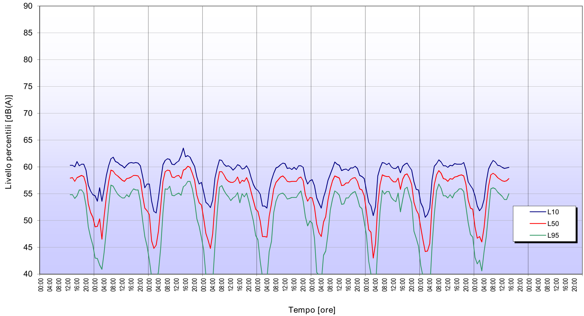
Punto PS1 GENOVA - Evoluzione temporale del segnale rilevato dal 28/05/2013 al 06/06/2013
