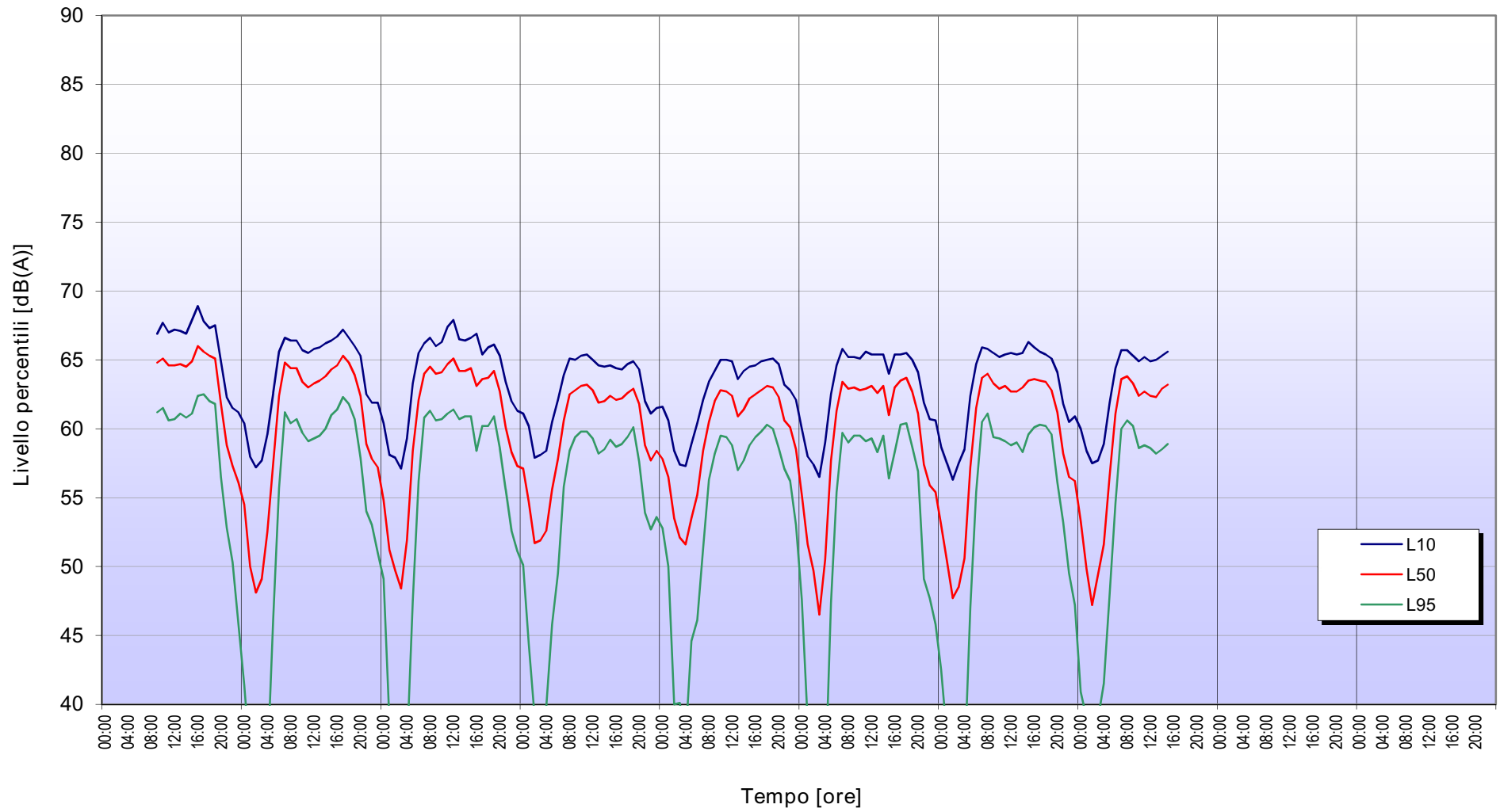
Punto PS3 GENOVA - Evoluzione temporale del segnale rilevato dal 29/05/2013 al 07/06/2013
