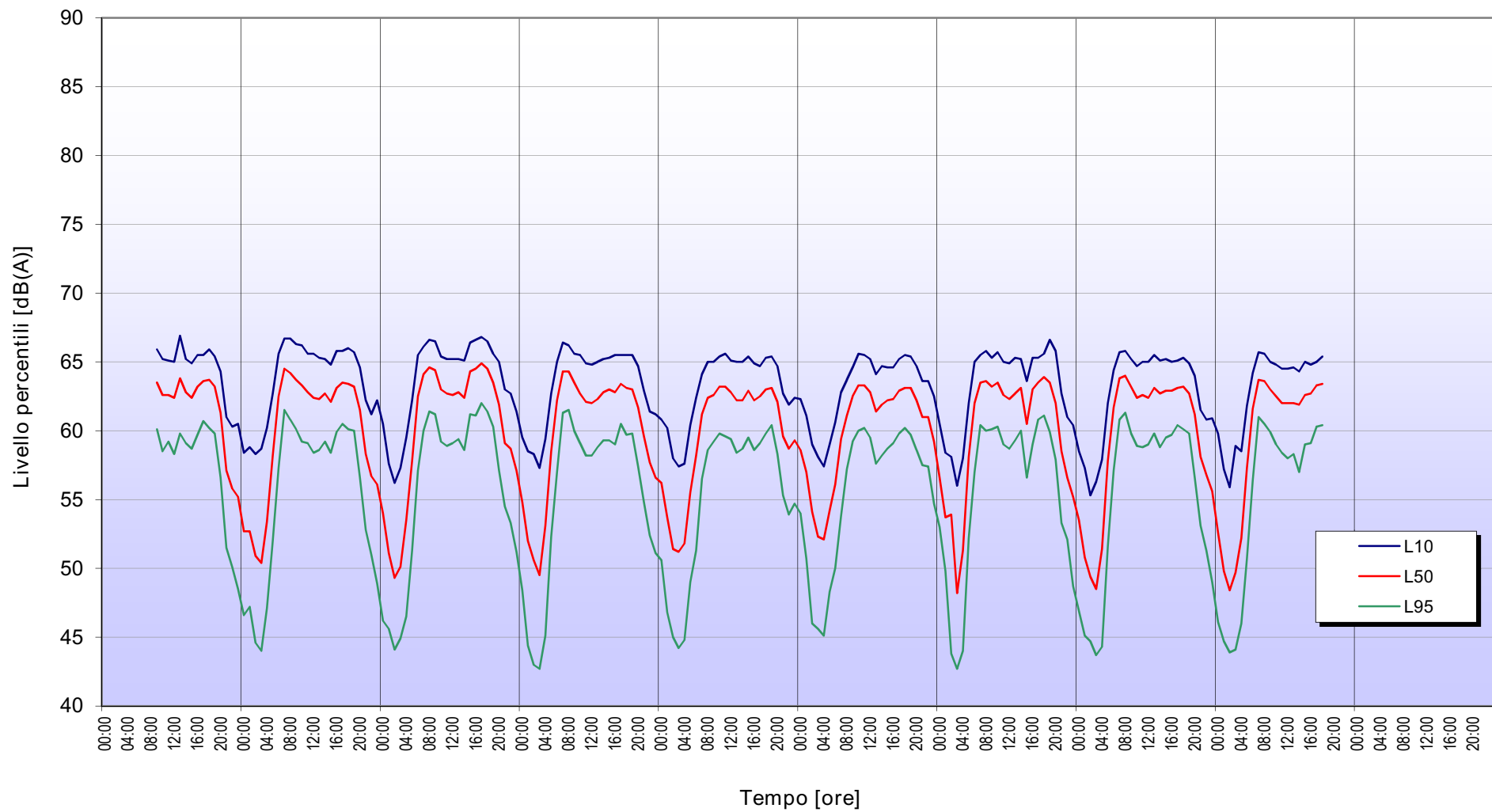
Punto PSR GENOVA - Evoluzione temporale del segnale rilevato dal 28/05/2013 al 06/06/2013
