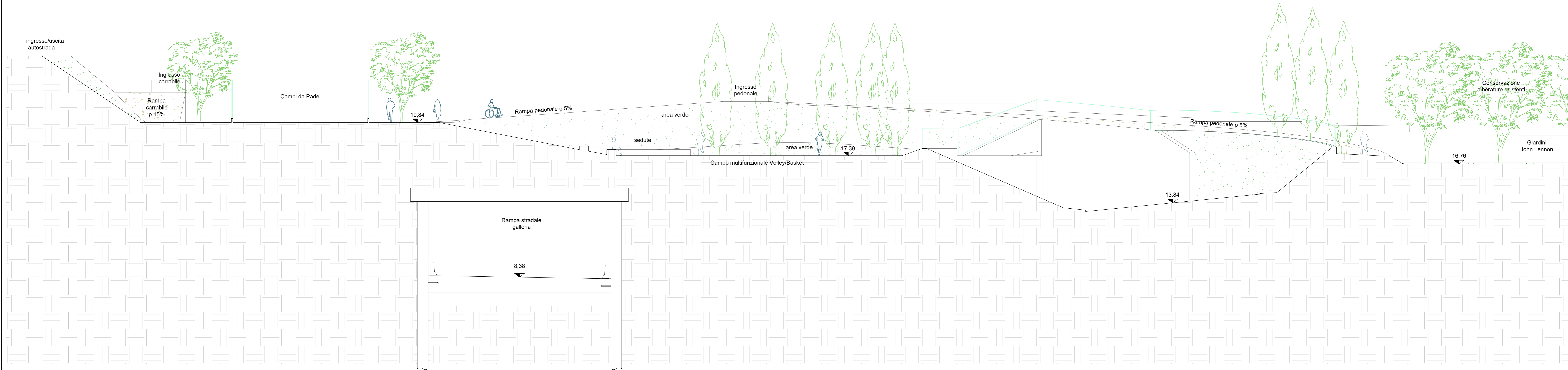
SEZIONE A-A'
