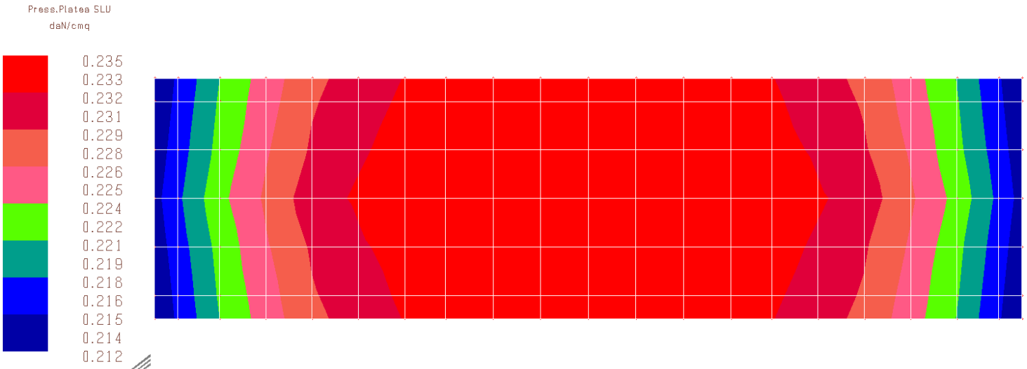
Involuppo delle pressioni sul terreno allo SLU
