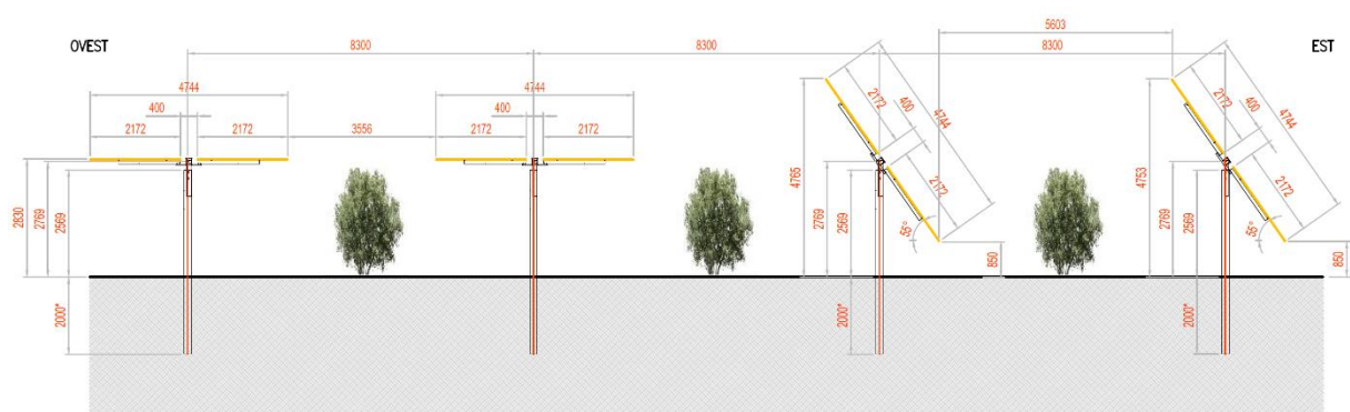
Figura 3.11: Tipologico – Vista Planimetrica dell'impianto Olivicolo
