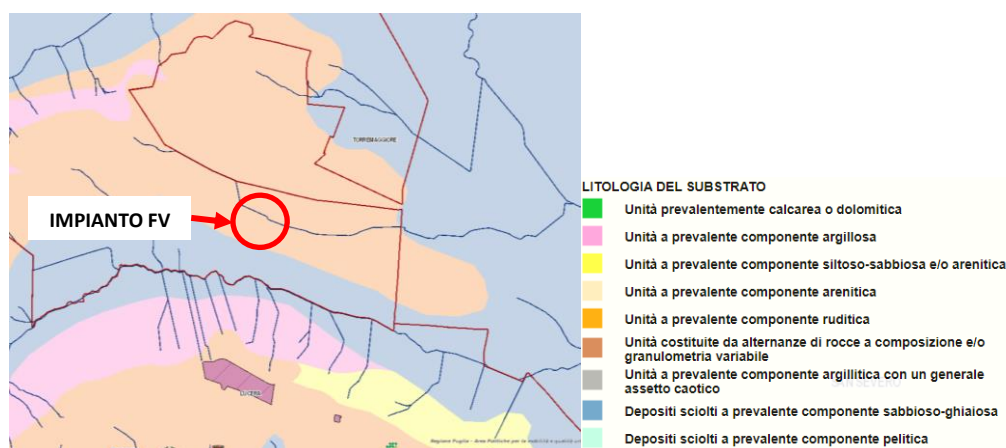
Figura 2.9: Stralcio carta idrogeomorfologica della Regione Puglia (modificata).
