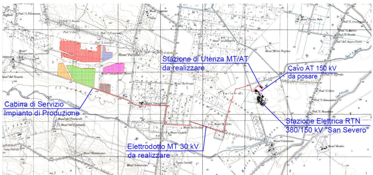
Figura 3.7: In rosso il percorso di connessione dal campo FV alla cabina di trasformazione
