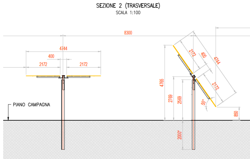
Figura 3.2: Particolare strutture di sostegno moduli
