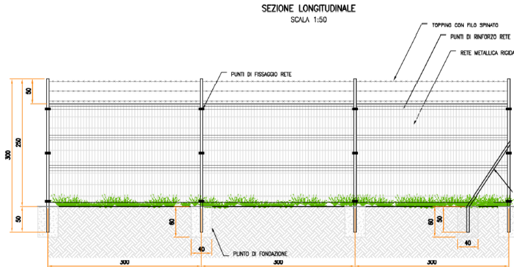
Figura 3.4: Particolare recinzione
