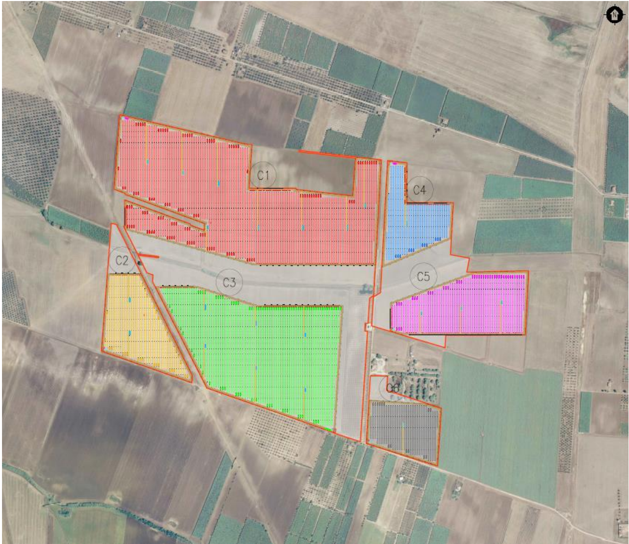
Figura 3.1: Layout di progetto
