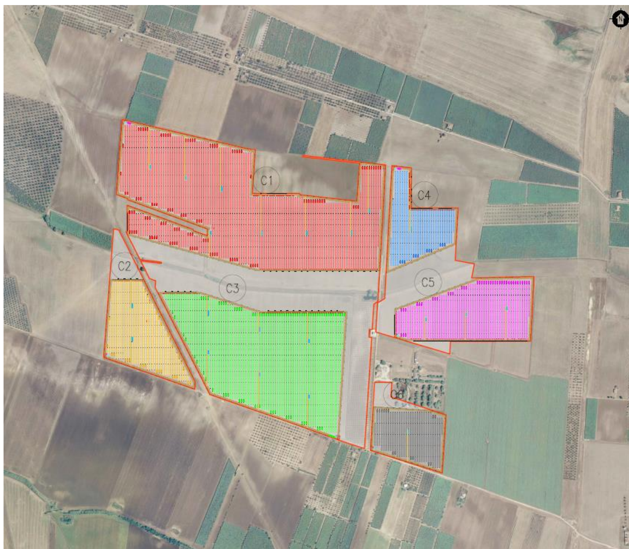
Figura 1.3: Layout di progetto
