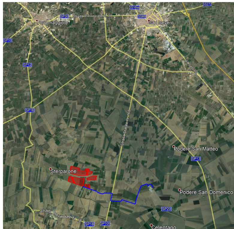
Figura 1.1: Localizzazione dell'area di intervento (rosso) e tracciato cavidotto AT (blu)
