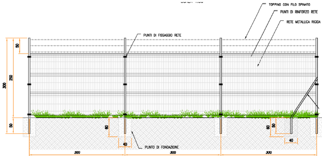
Figura 4.6: Particolare recinzione
