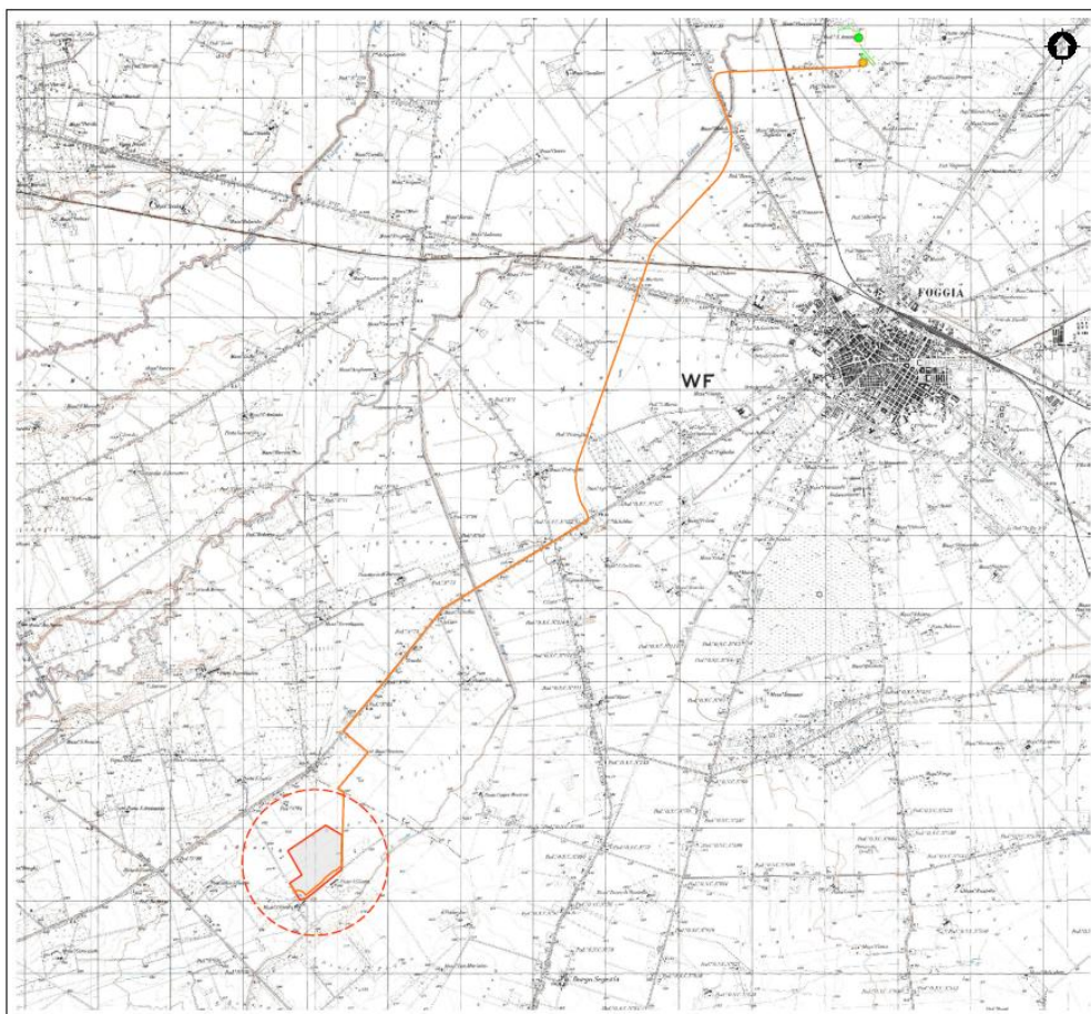
Figura 2.1: Localizzazione dell'area di intervento (rosso: impianto; arancione: linea di connessione MT; verde: connessione AT)
