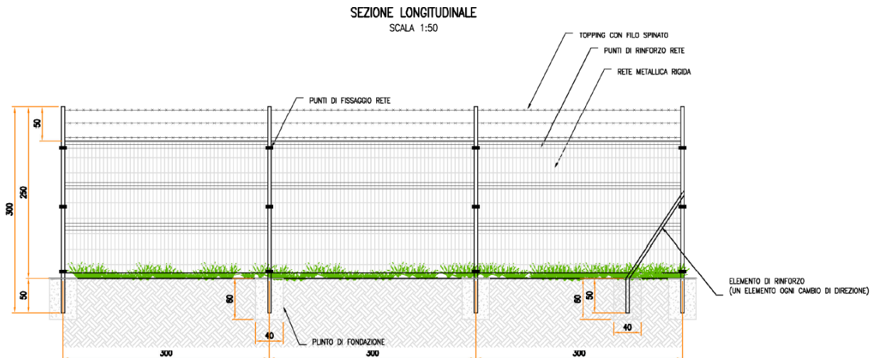
Figura 5.1: Tipico recinzione
