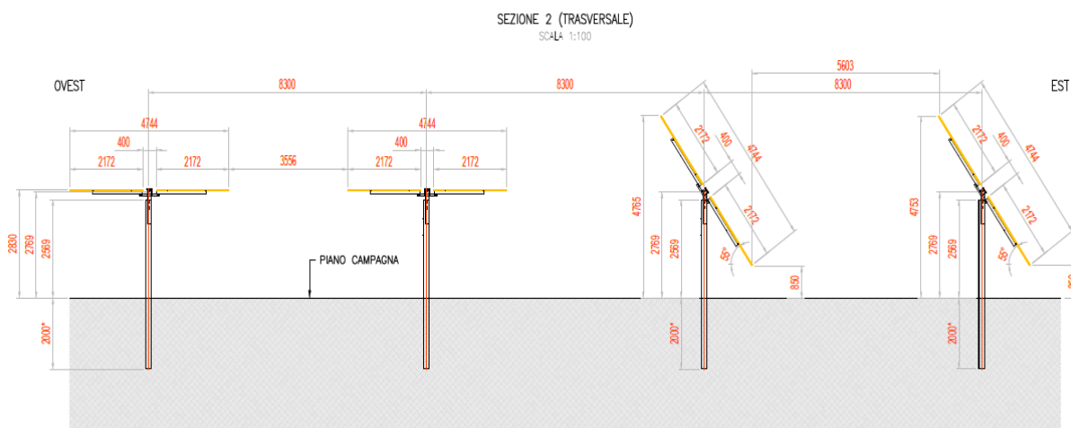
Particolare strutture sostegno moduli pannelli e distanze di campo
