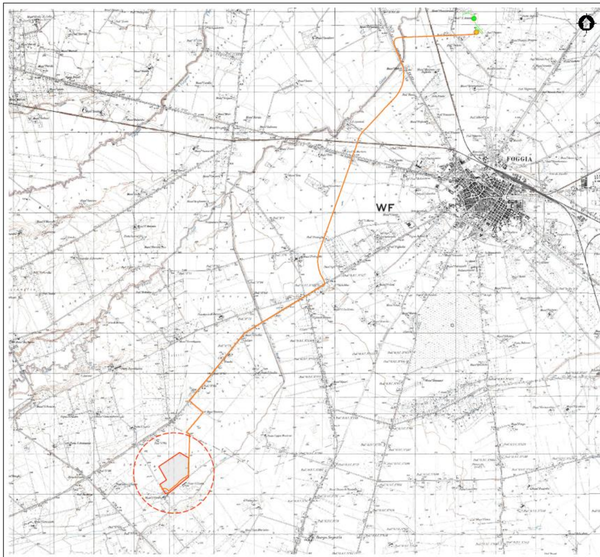
Figura 2.5: Localizzazione dell'area di intervento (rosso: impianto; verde: connessione)
