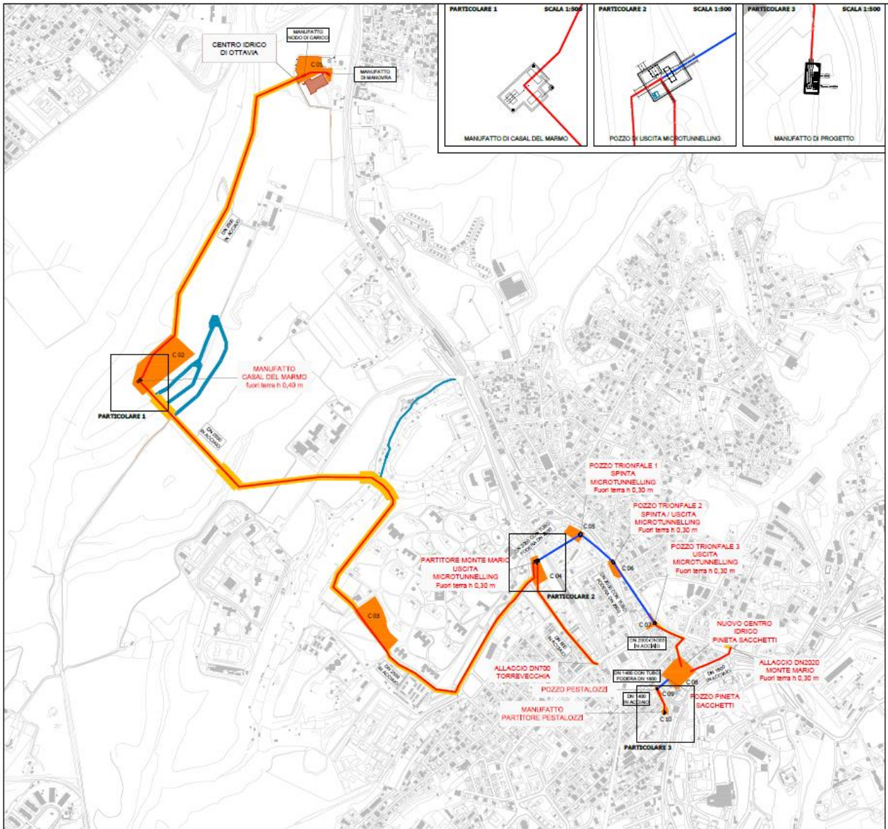
Figura 5-1 Planimetria generale delle aree di cantiere
