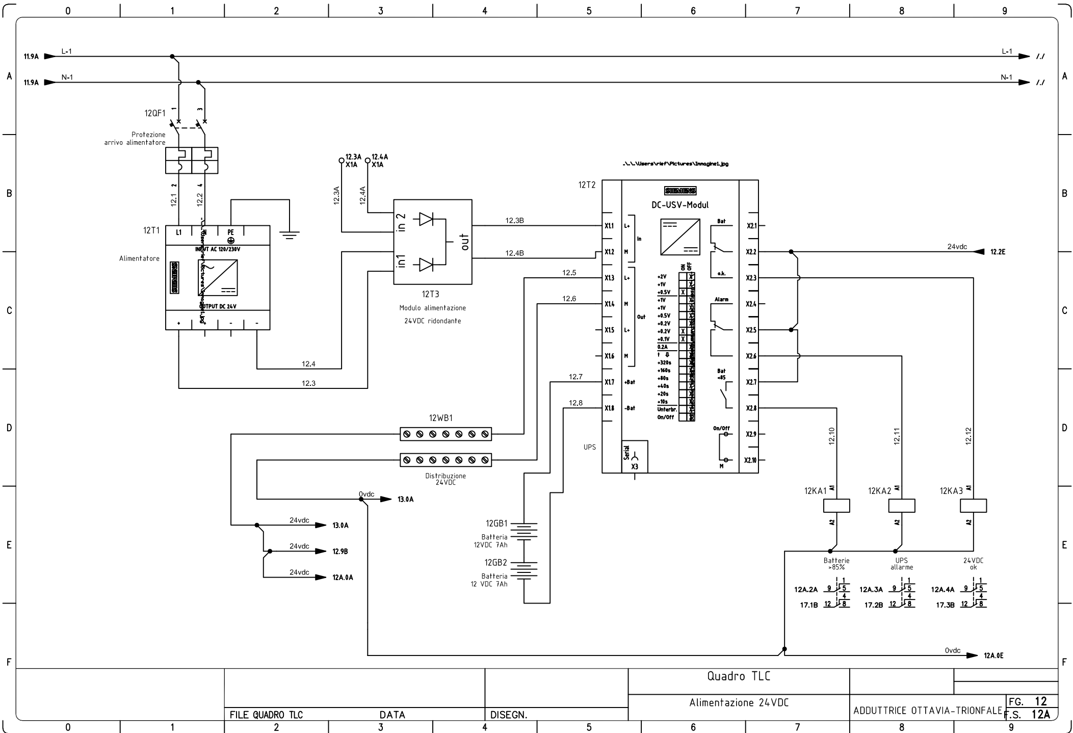
Annex 3 - Schema Quadro RTU
