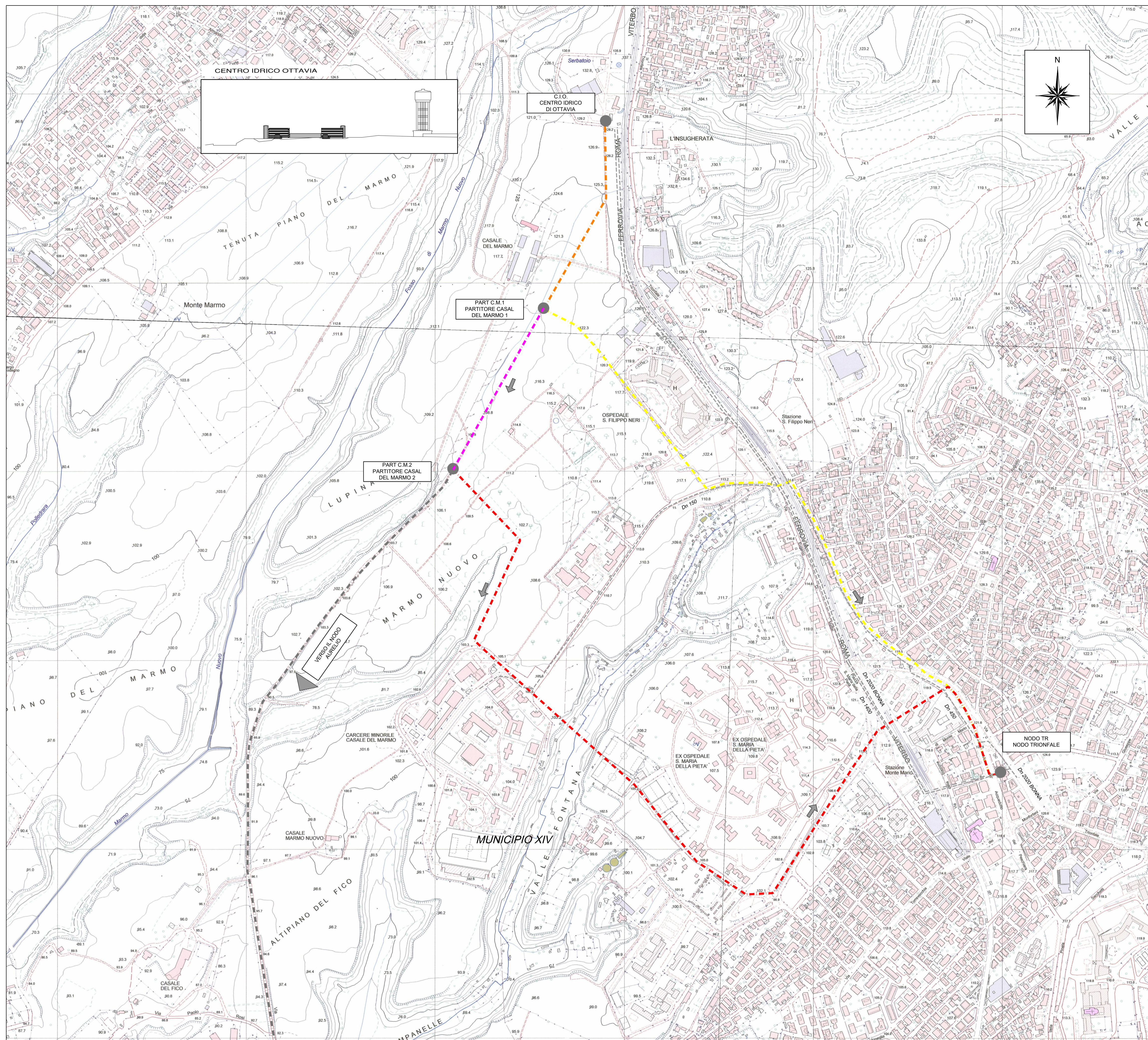
STRALCIO PLANIMETRICO - TRATTO 1 - SOLUZIONE TR1 TR2 - CENTRO IDRICO DI OTTAVIA - NODO TRIONFALE - SCALA 1:5000
