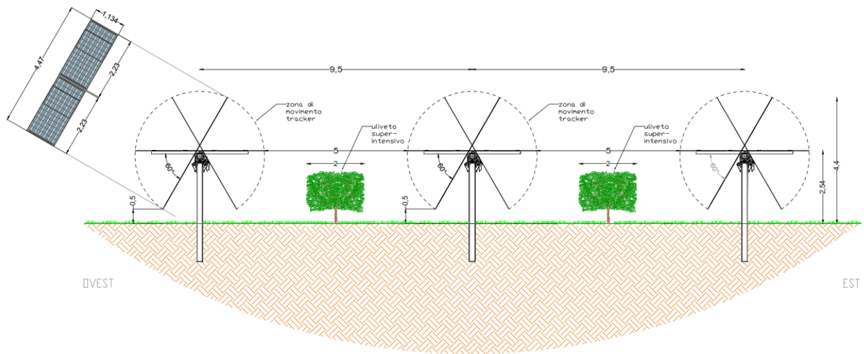
Fig. n°1 Sistema Agro-fotovoltaico
