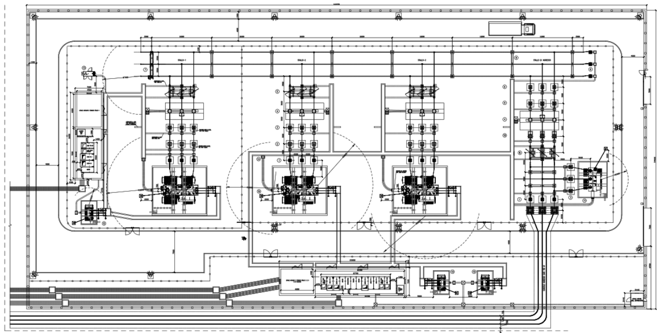
Fig. 9 Planimetria sottostazione utente
