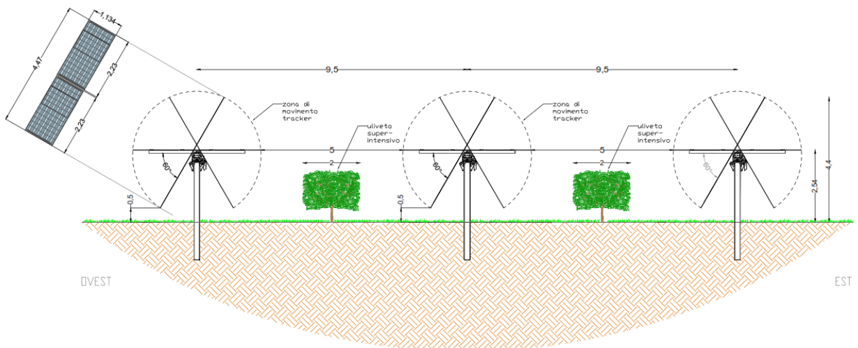
Fig. n°18 Pitch dei tracker
