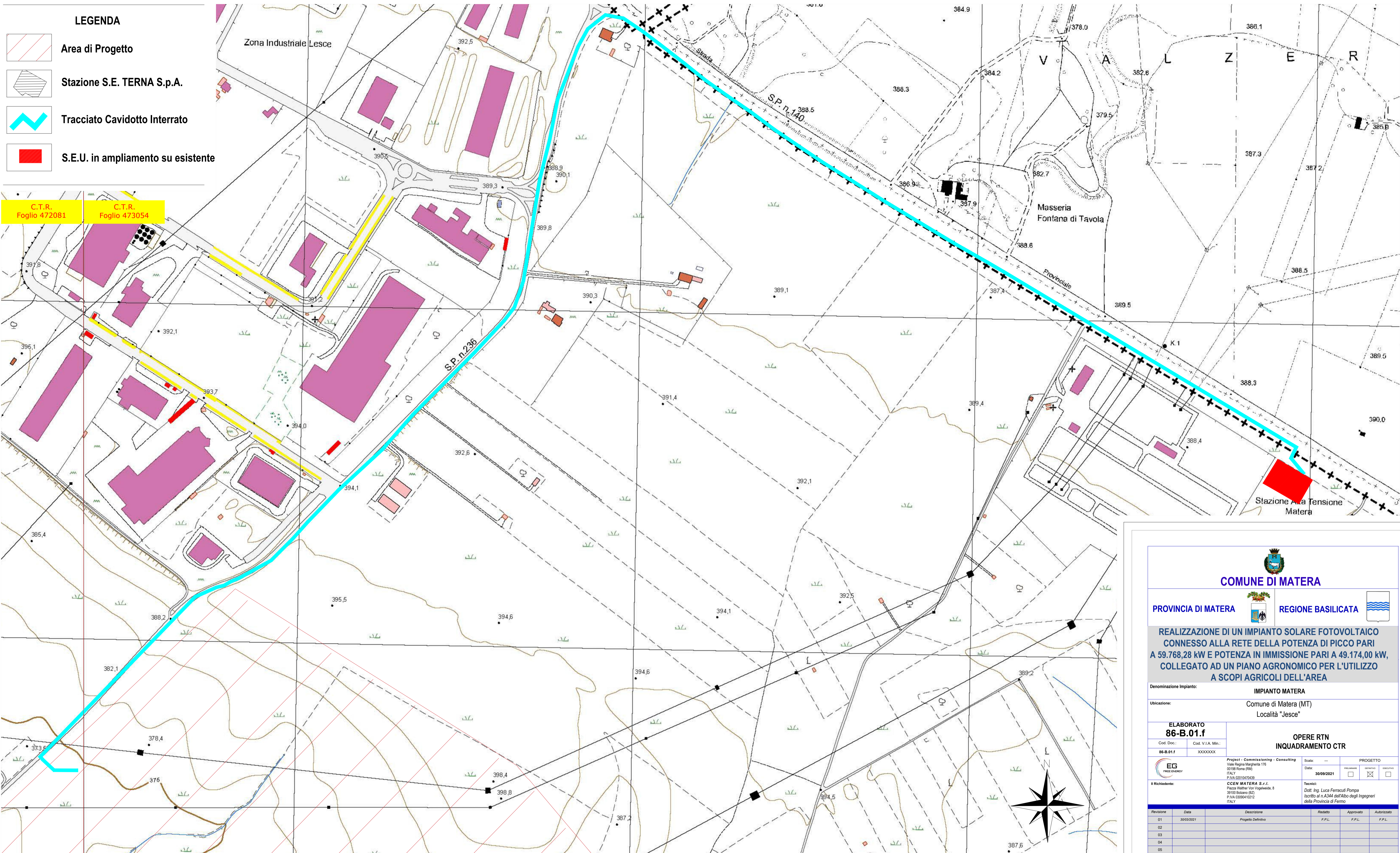
PLANIMETRIA CAVIDOTTO SU CARTA TECNICA REGIONALE Comune di MATERA (MT) - scala di rappresentazione 1:2.000 -
