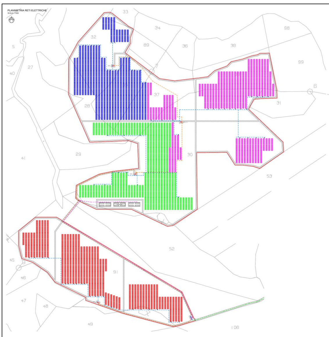
Figura 1 - Layout impianto
