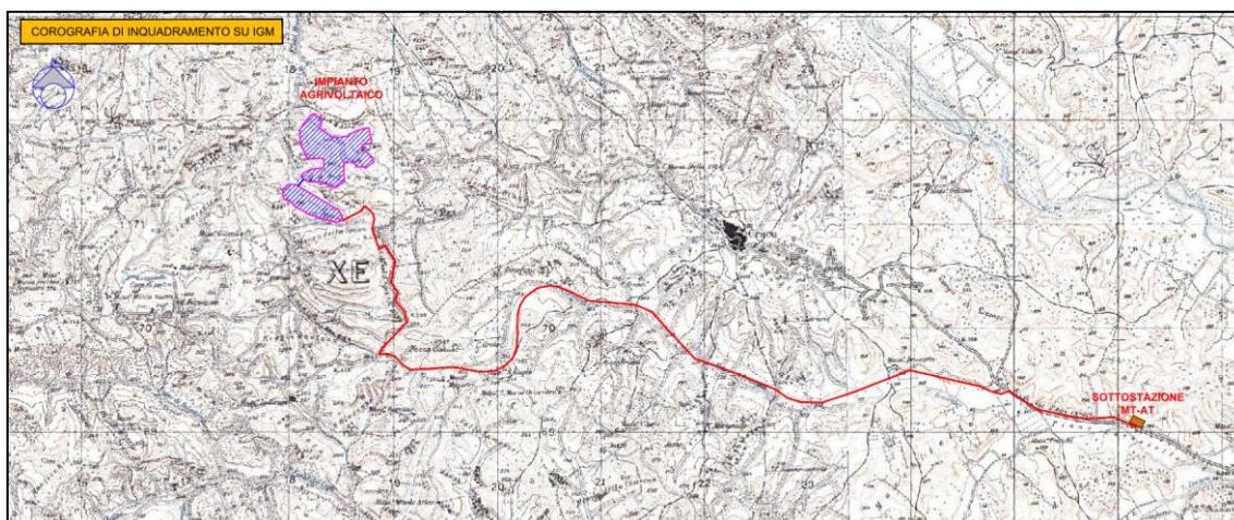
Figura 2 – Inquadramento impianto (Stralcio tavola G13909A01 – A12a1-2 Corografia di inquadramento su IGM)
