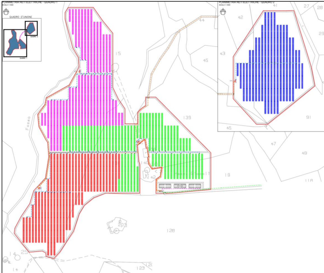
Figura 1 - Planimetria impianto agrivoltaico
