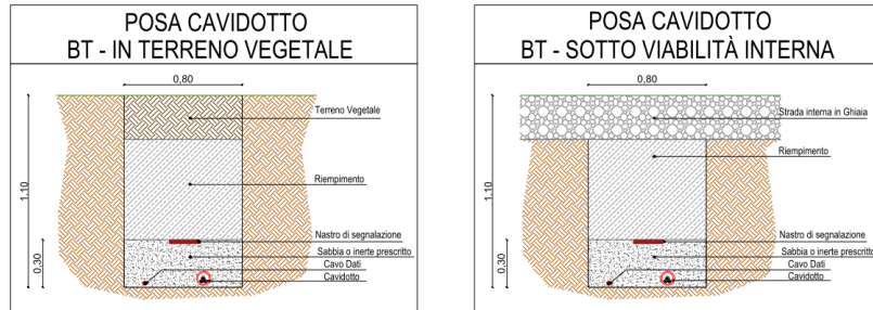
Figura 44 - Sezioni di scavo dei cavidotti
