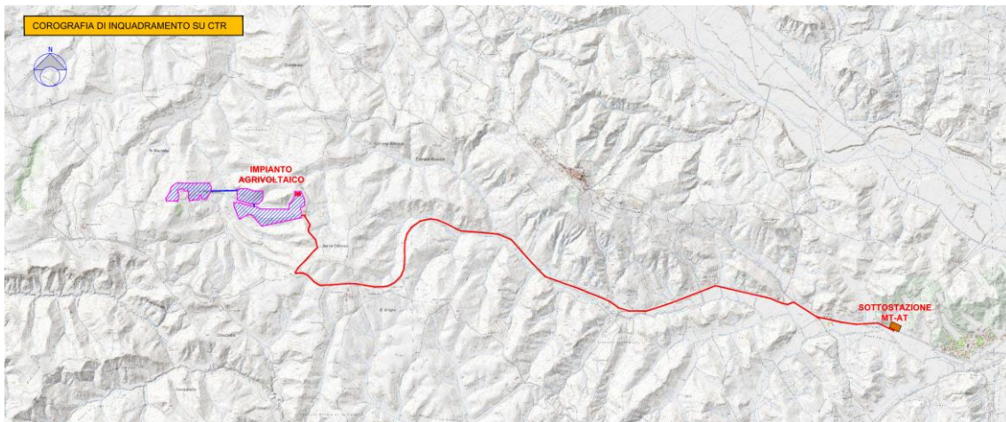
Figura 2 - Stralcio della corografia generale di progetto
