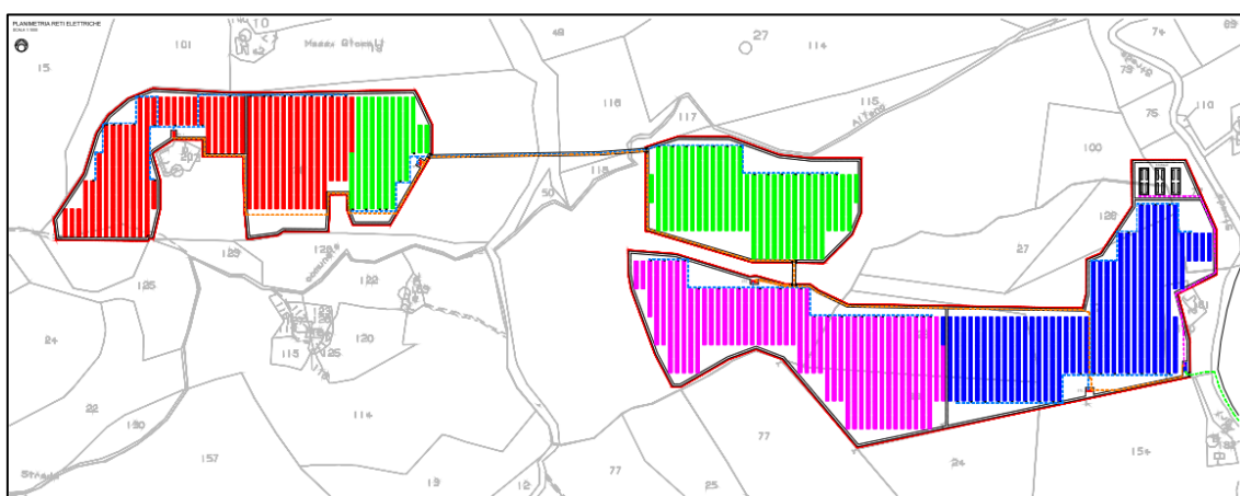
Figura 1 - Layout impianto
