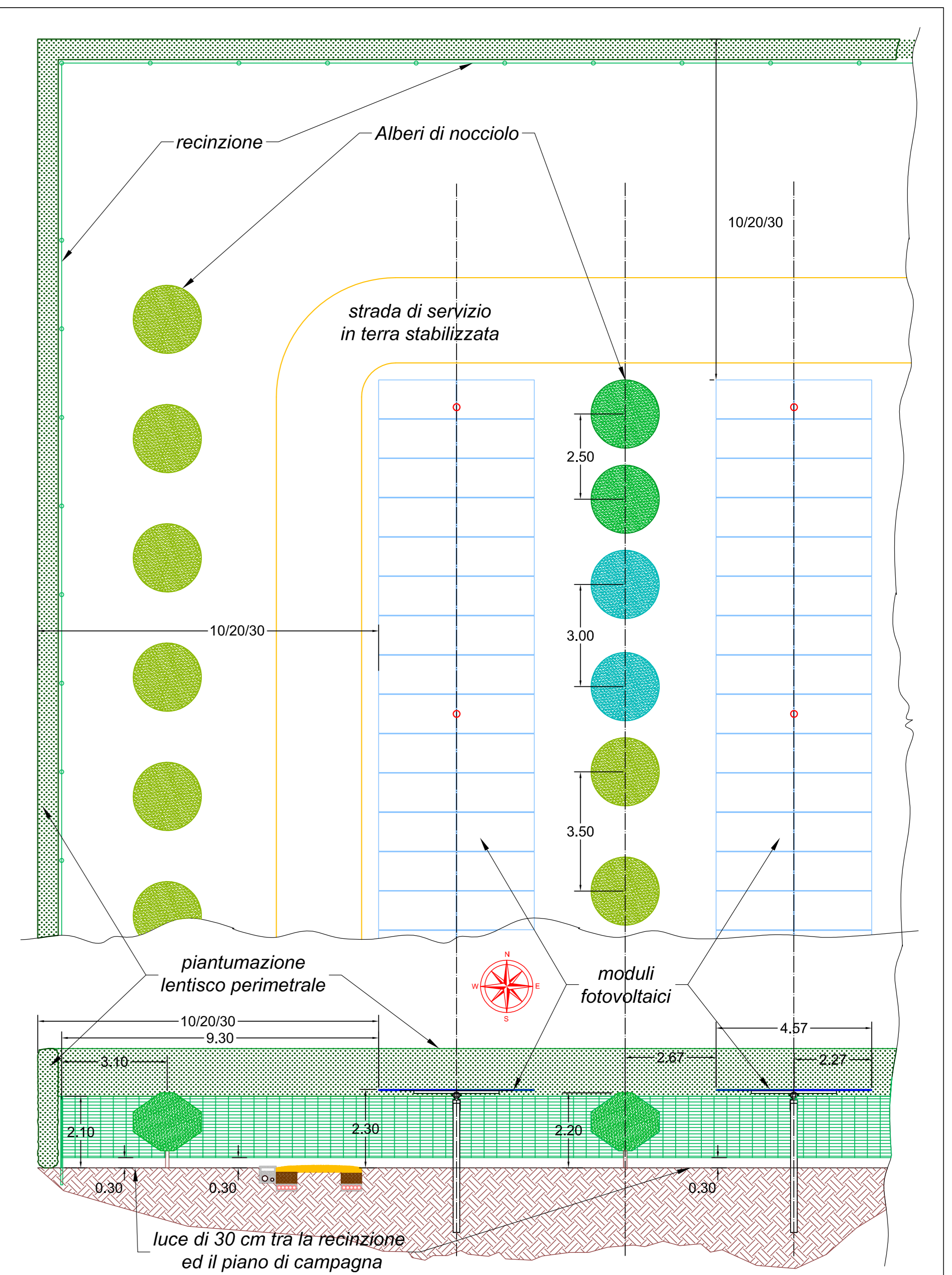
Particolare "consociazione" impianto FV e arboricoltura e piantumazione perimetrale di Lentisco Scala 1: 1.00
