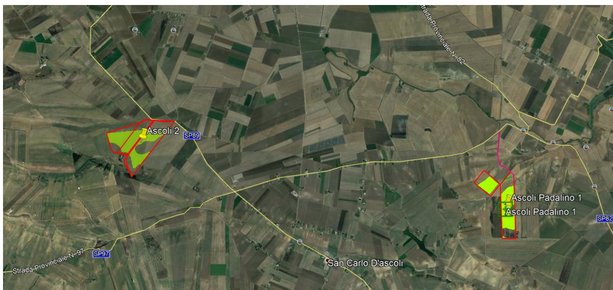
Area di progetto dell'impianto fotovoltaico su ortofoto.
