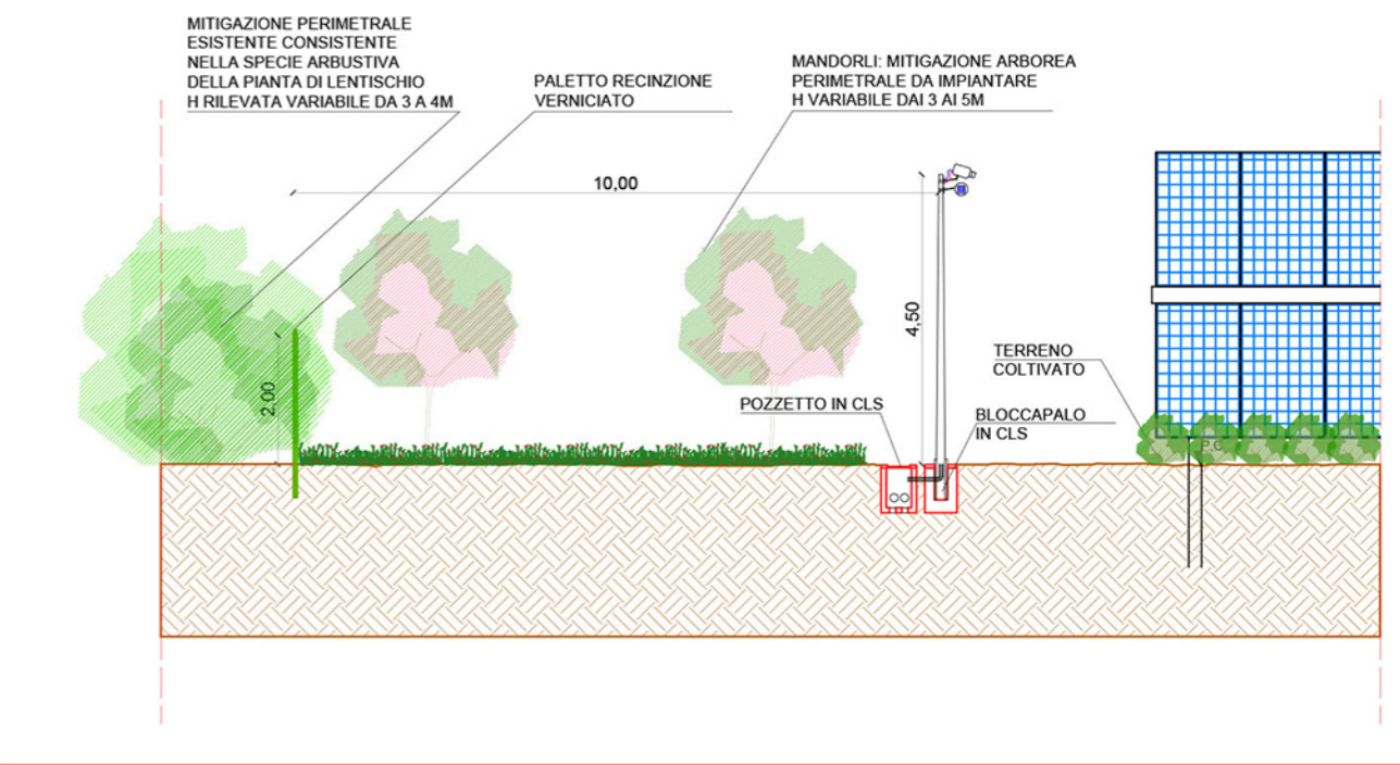
RAPPRESETAZIONE MITIGAZIONE SEZIONE TRASVERSALE
