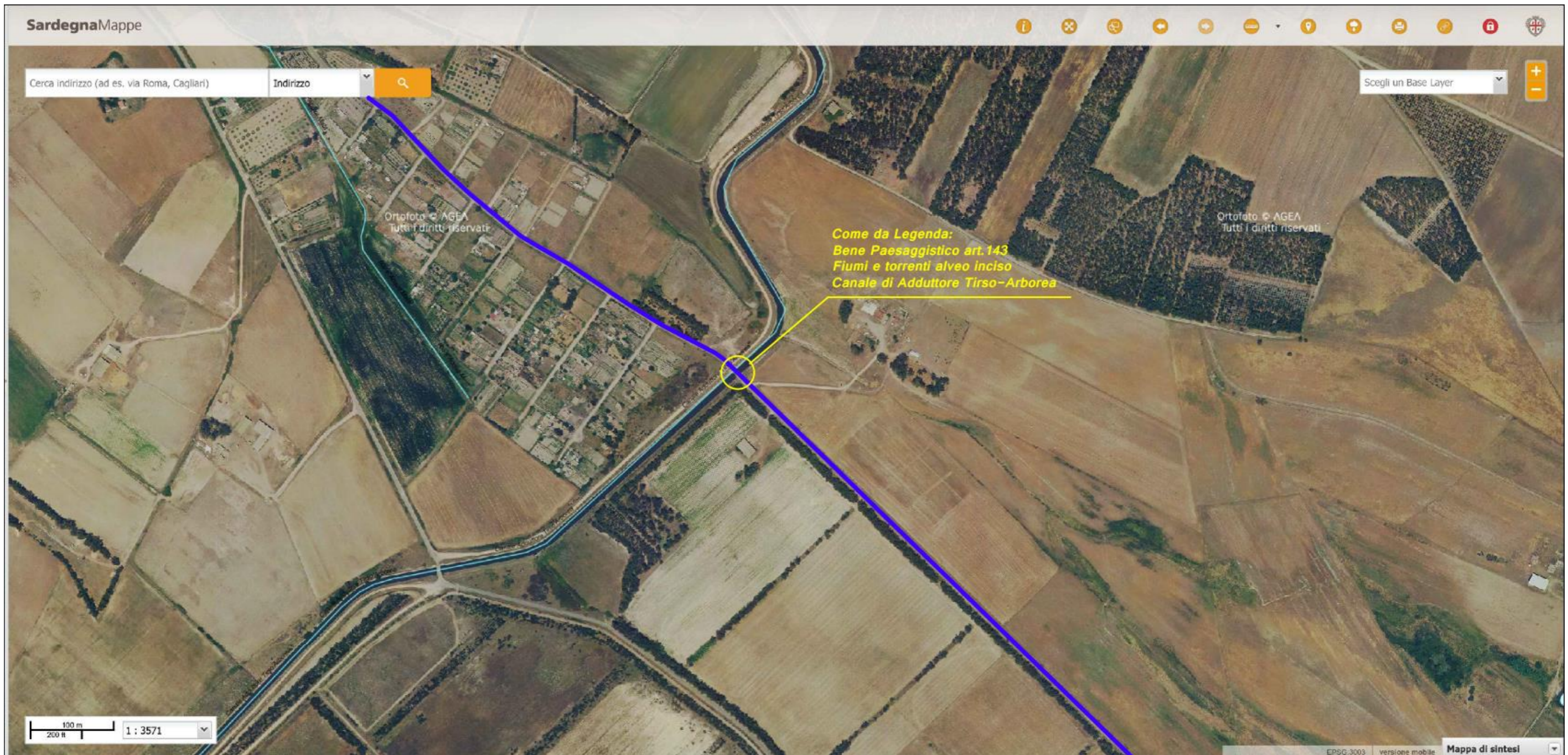
Dettaglio 3: Tratto cavidotto su strada comunale, interferenza con il canale Adduttore Tirso-Arborea, risoluzione interferenza a mezzo T.O.C. (Trivellazioni Orizzontali Controllate)
