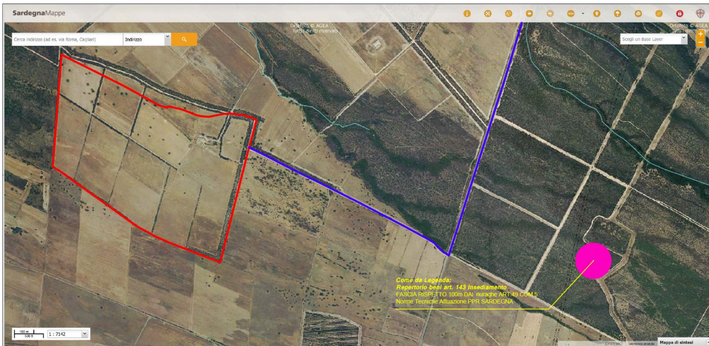
Dettaglio 1: Area impianto e tratto cavidotto su SP68, nessuna interferenza
