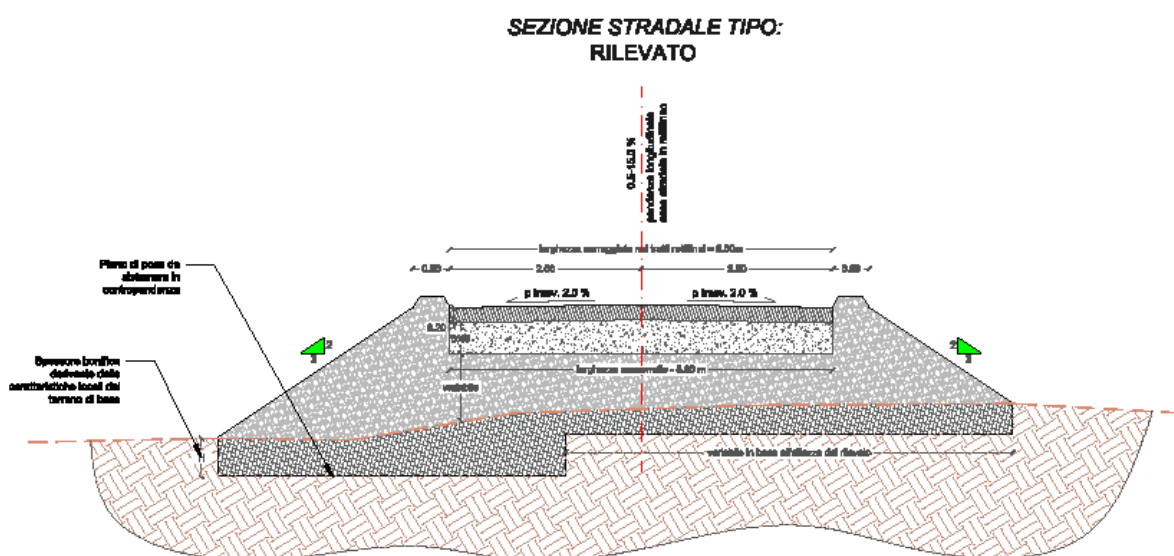
Figura zz: sezione stradale tipo in rilevato all'interno del parco eolico
