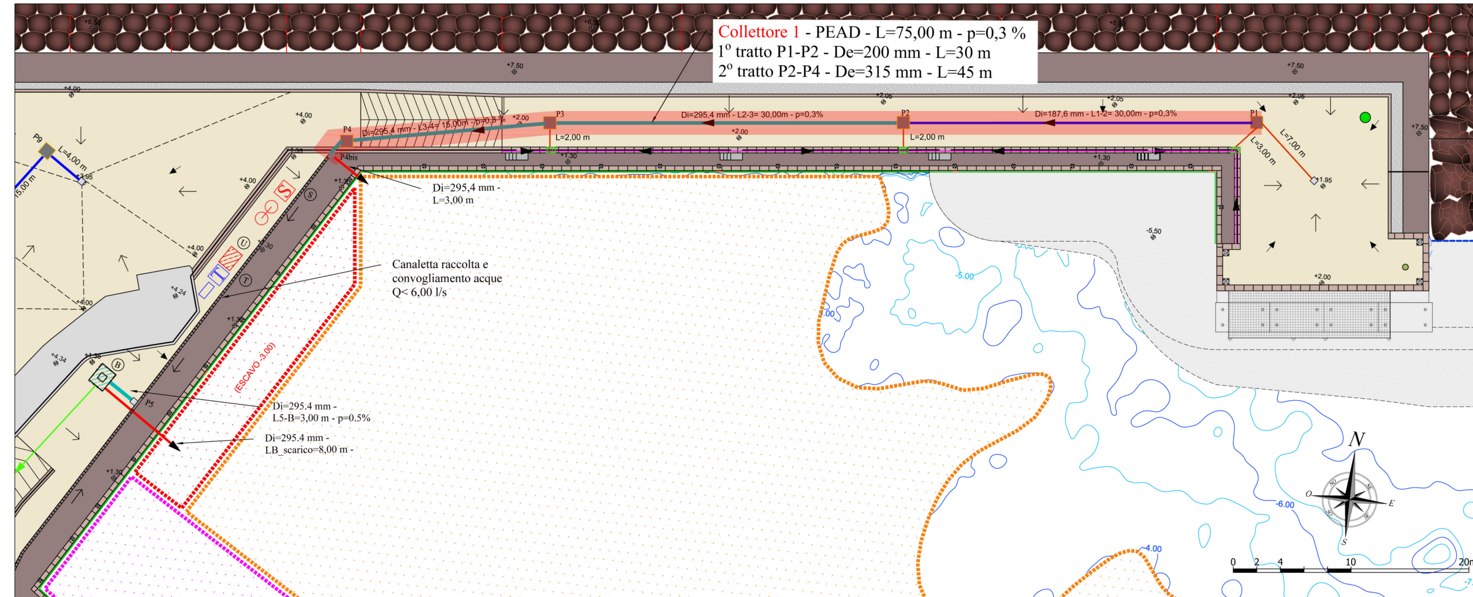
Planimetria collettore 1 - Scala 1:200
