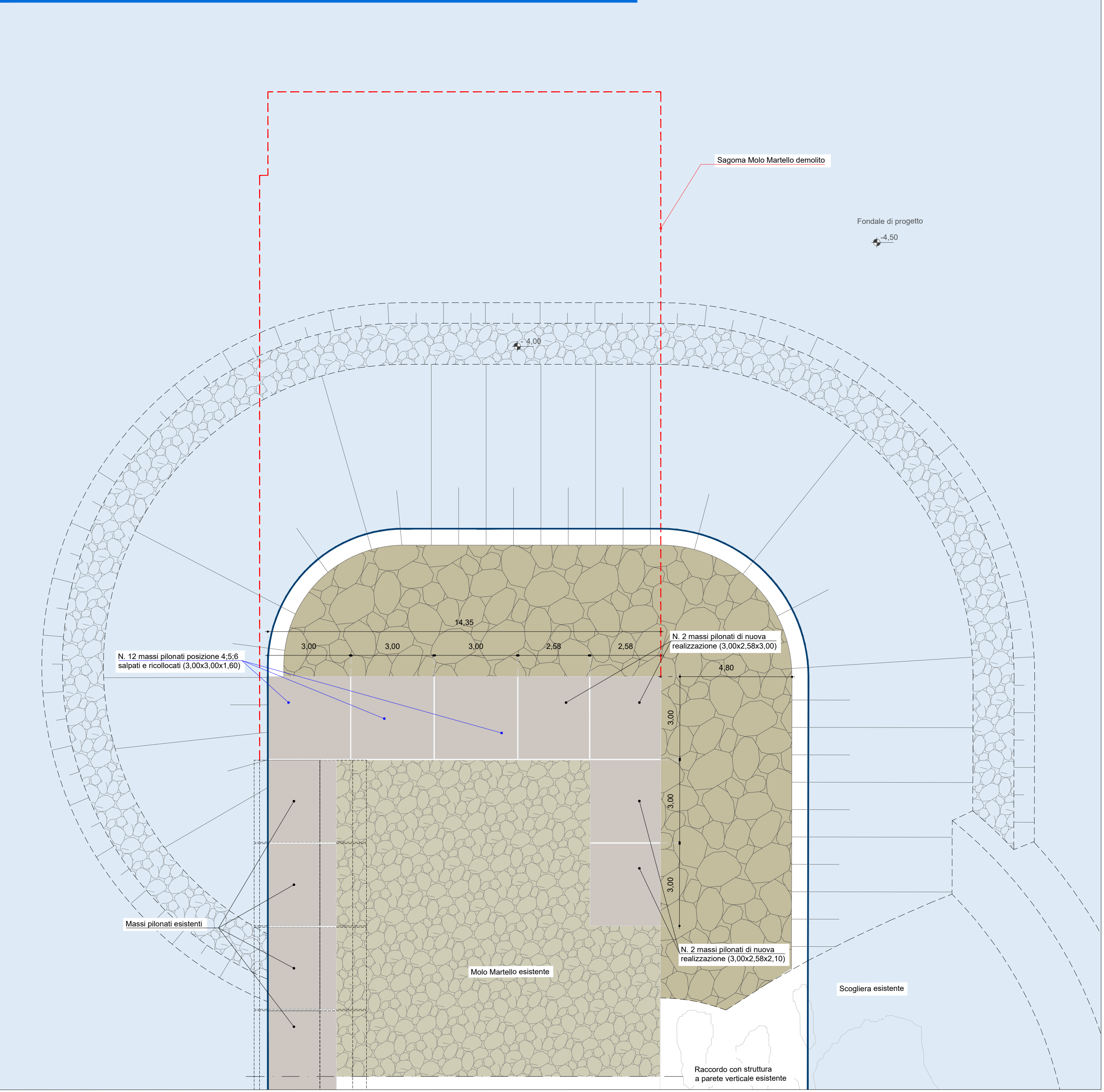
STRALCIO PLANIMETRICO - RICOSTRUZIONE PILONATI TESTATA MOLO MARTELLLO - QUOTA + 0,40 m - scala 1:100
