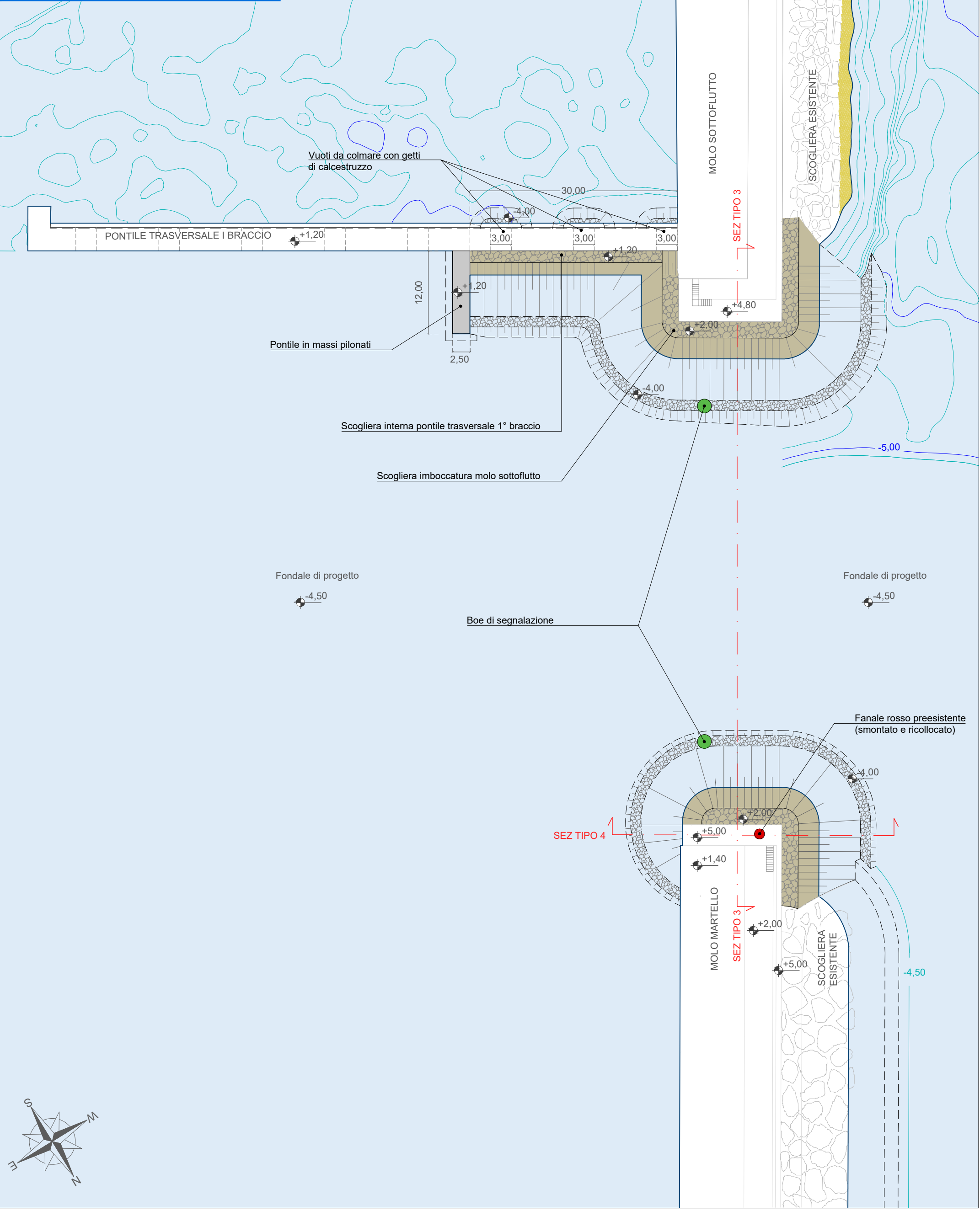
STRALCIO PLANIMETRICO - scala 1:500
