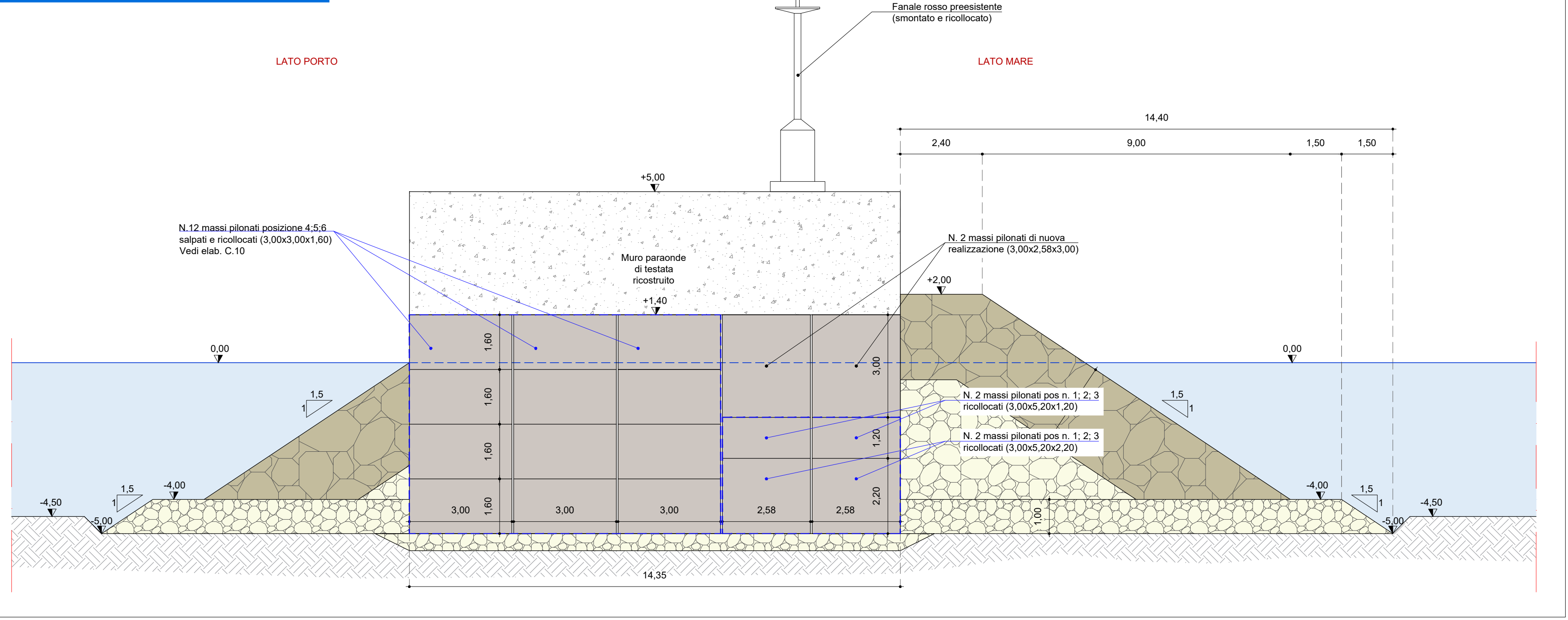
SEZIONE TIPO 4 MOLO MARTELLLO - scala 1:100
