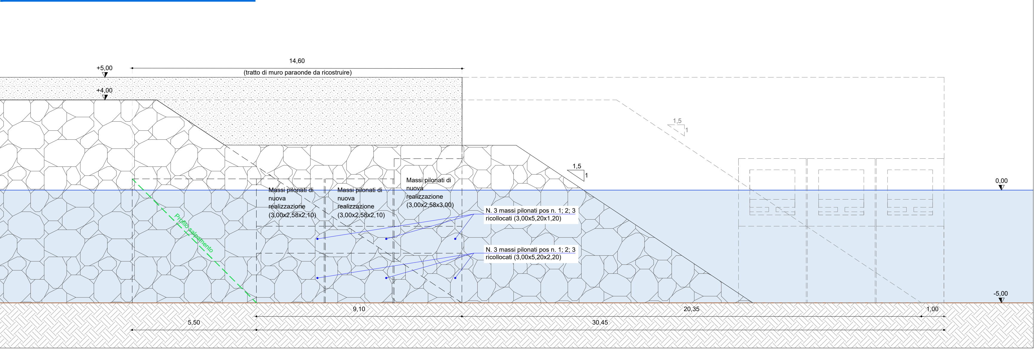
SEZIONE TIPO 4 MOLO MARTELLLO - scala 1:100
