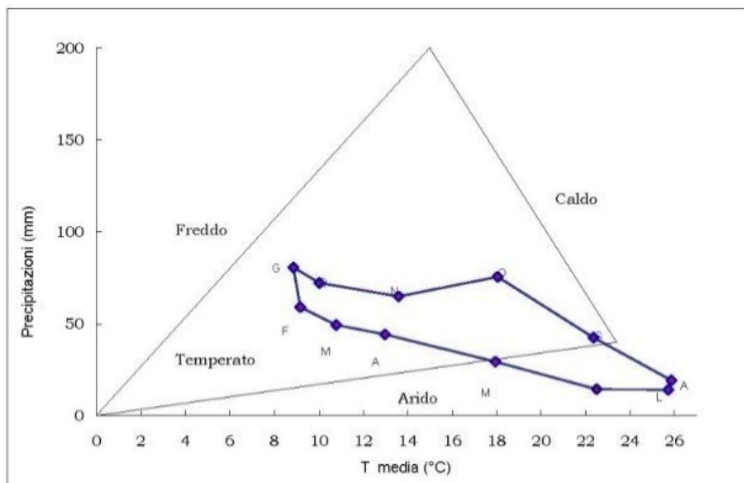
Figura 2: Diagramma chimogrammi di Peguy Agrigento - "Climatologia della Sicilia"
