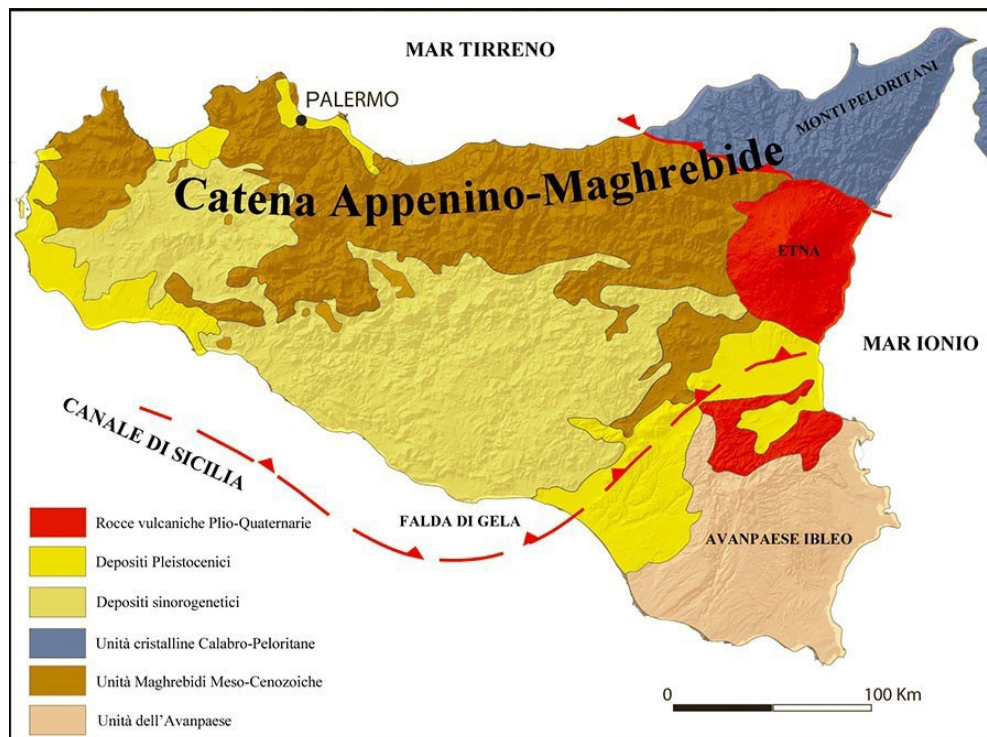
Figura 4: Schema tettonico Sicilia
