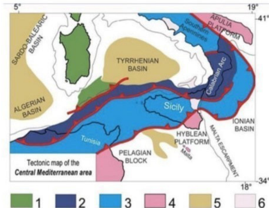
Figura 3: Schema tettonico del Mediterraneo centrale (Catalano et al., 2001). 1) Corsica-Sardegna; 2) Arco Kabili-Peloritano_Calabro; 3) Unità Appenninico-Maghrebide e dell'avampese deformato; 4) avampese ed avampese poco deformato; 5) aree in estensione; 6) vulcaniti plio-quaternarie
