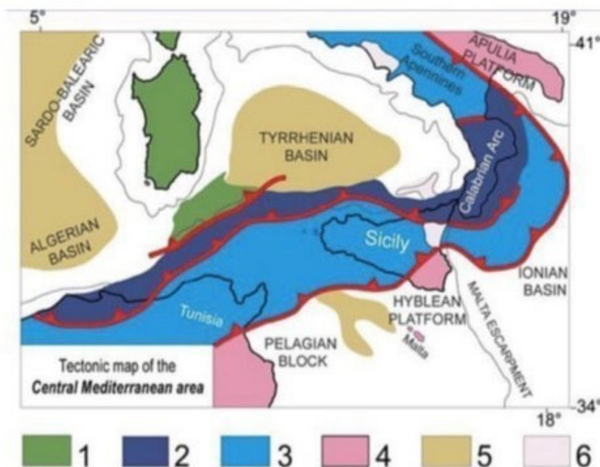
Figura 3: Schema tettonico del Mediterraneo centrale (Catalano et al., 2001). 1)
