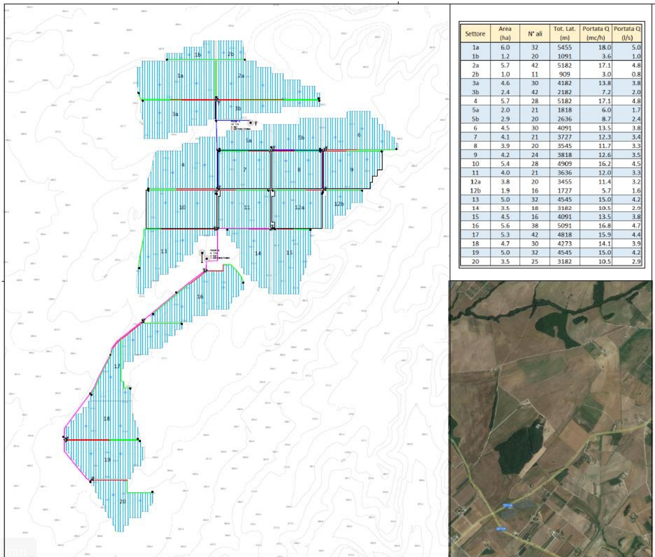
Figura 11. Dettaglio layout impianto di irrigazione
