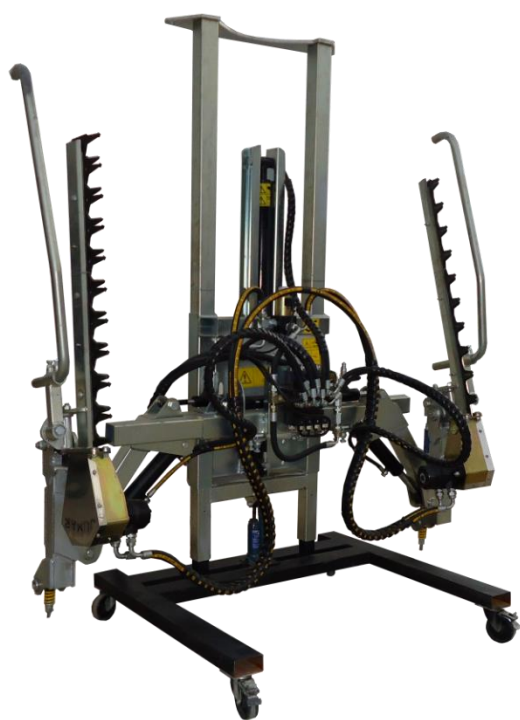
Figura 19. Raccorciatrice di rami bassi. Mod. Duplex (sinistra). Indicazione dell'area di pulizia rami bassi (destra)
