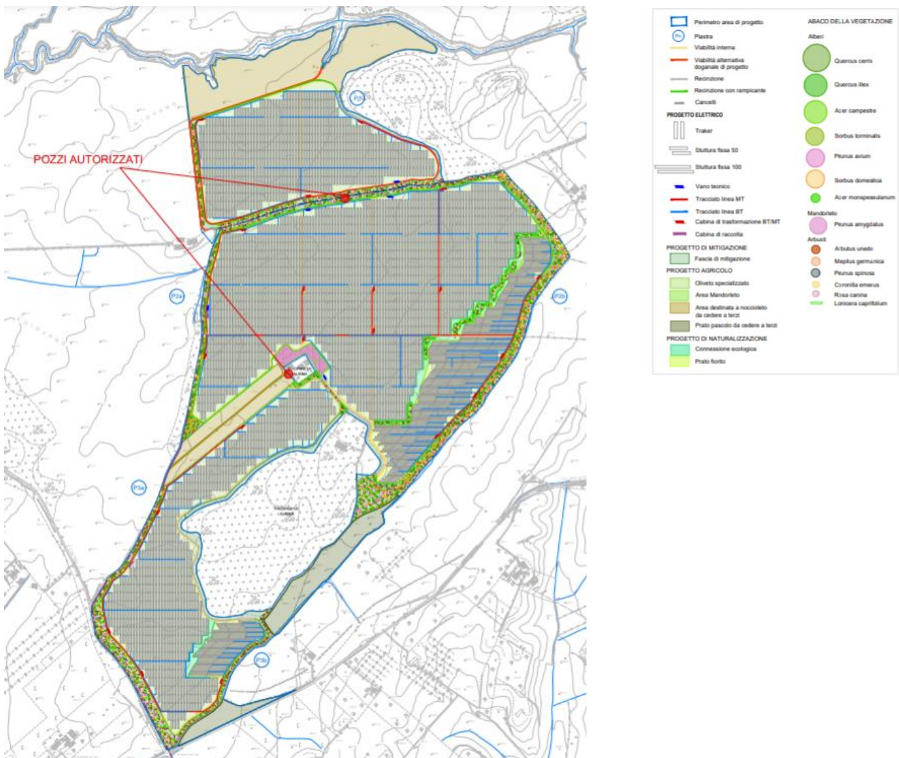
Figura 7. Descrizione del layout agri-voltaico del progetto
