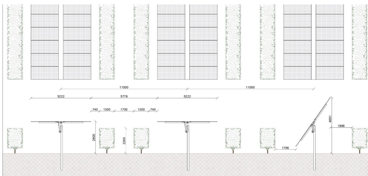
Figura 12. Dettaglio layout impianto agri-voltaico
