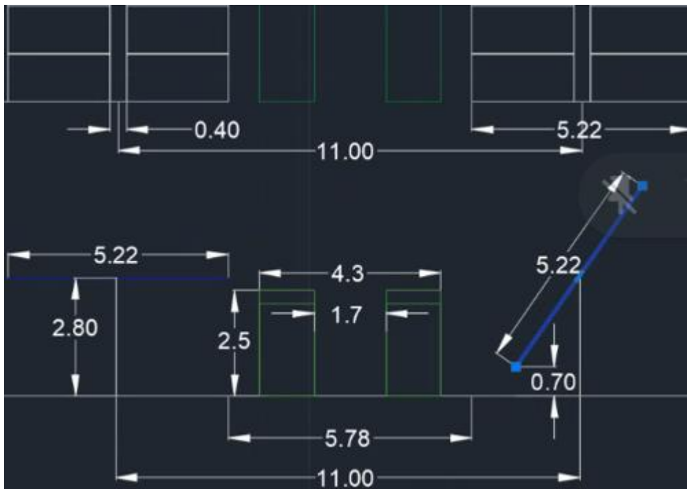
Figura 9. Descrizione del sesto di impianto e dell'interfila
