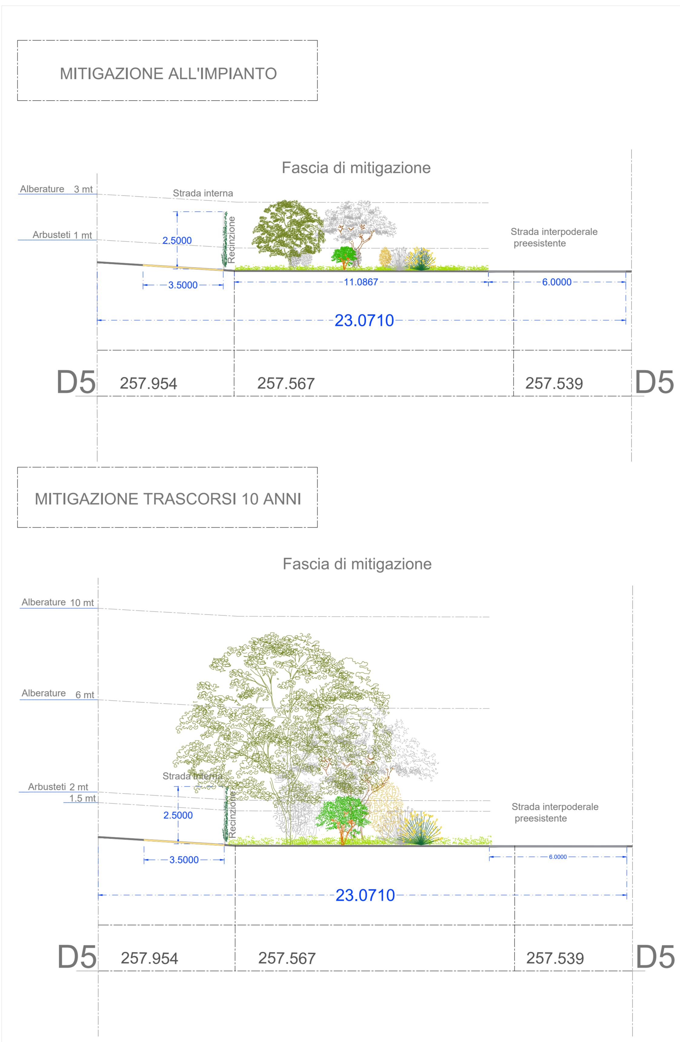
Dettaglio D5 Scala 1:100
