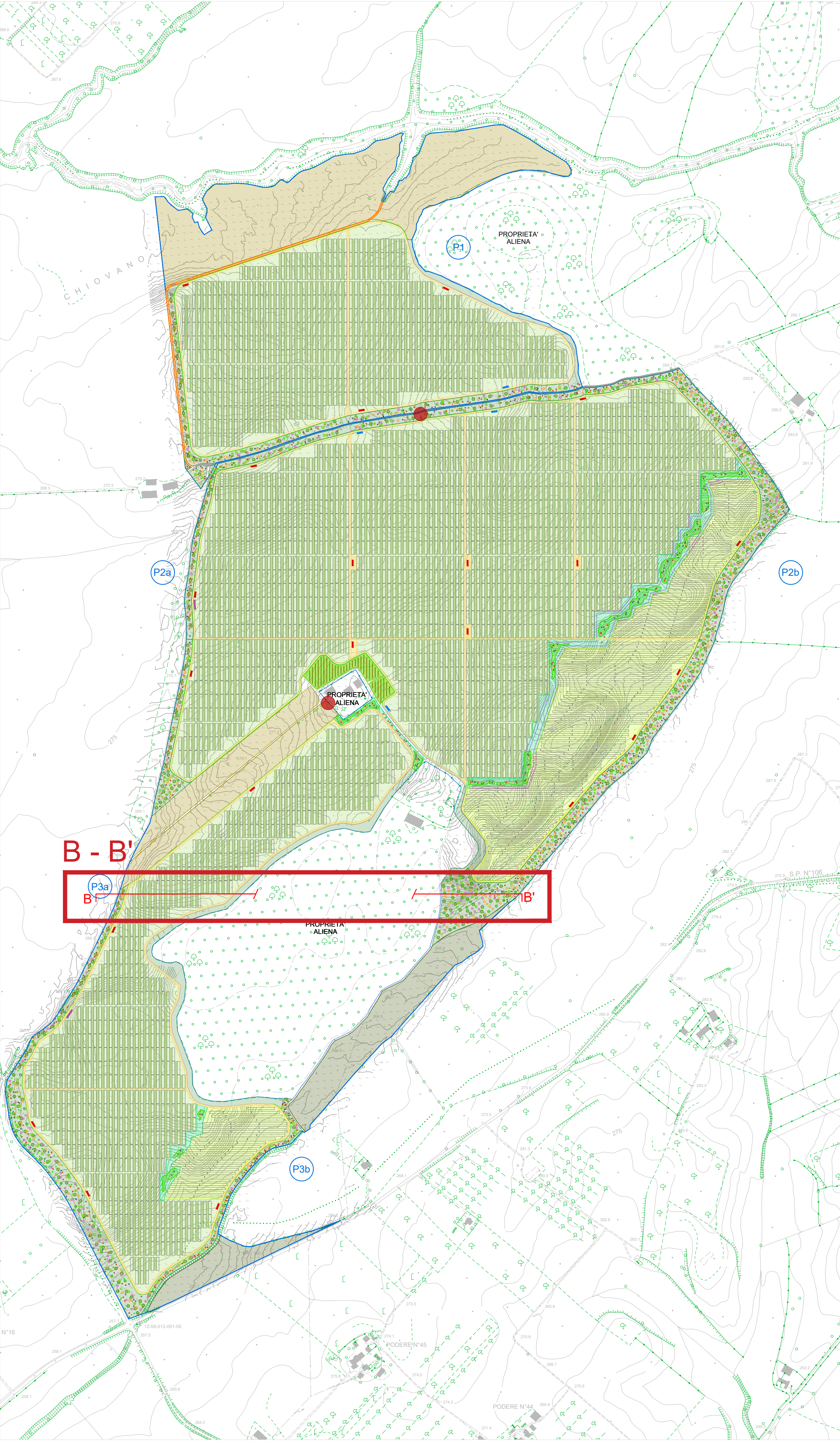
Sezione stato di fatto e stato di progetto B - B' scala 1:5.000
