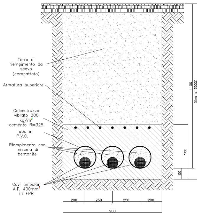
TIPOICO CAVIDOTTO A.T. INTERRATI POSA INTERRATA IN ATTRAVERSAMENTO NELLA CONFIGURAZIONE IN PIANO
