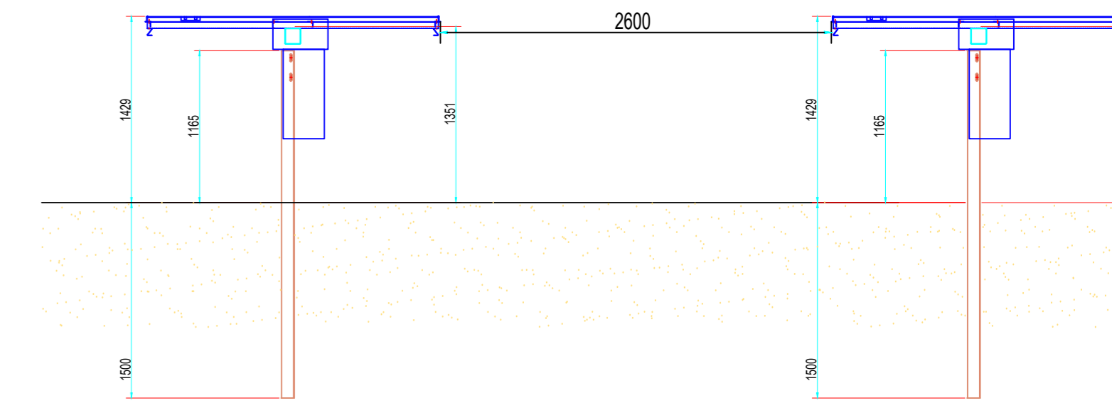
Inseguitore monoassiale - Vista laterale con inclinazione a 0°
