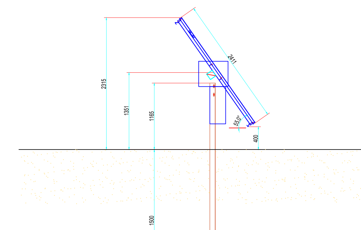
Inseguitore monoassiale - Vista laterale con inclinazione a 55°
