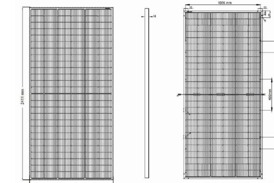
MODULO FOTOVOLTAICO - JINKO SOLAR JKM580M-7RL4-TV
