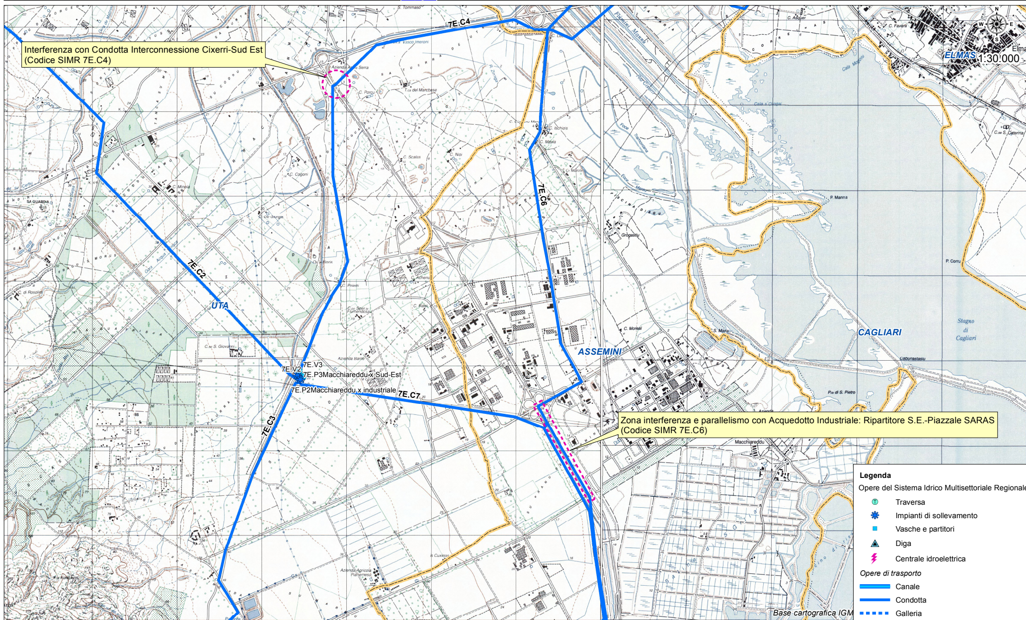
Opere del Sistema idrico Multisetoriale Regionale (SIMR) gestite dall'Enas. Individuazione interferenze cavidotto terrestre HVAC 245kV impianto eolico offshore "SARDEGNA 1"
