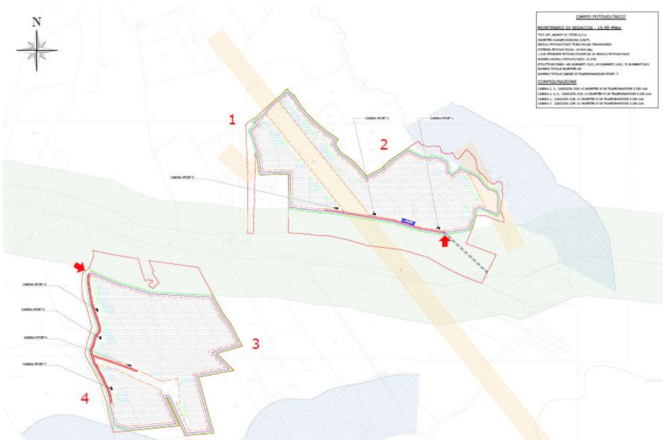
LAY-OUT IMPIANTO
