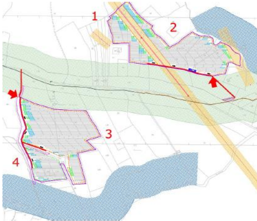
LAY-OUT IMPIANTO
