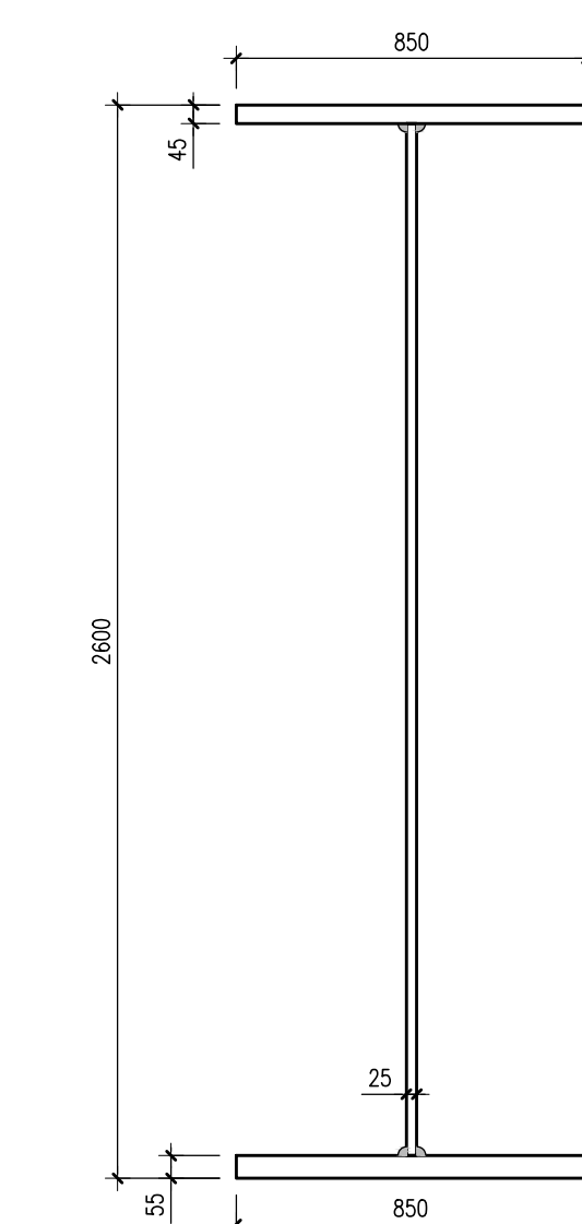
SEZIONE CONCIO 2
