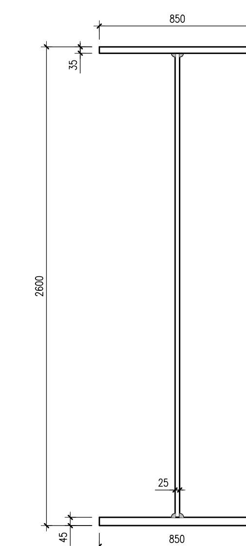
SEZIONE CONCIO 1
