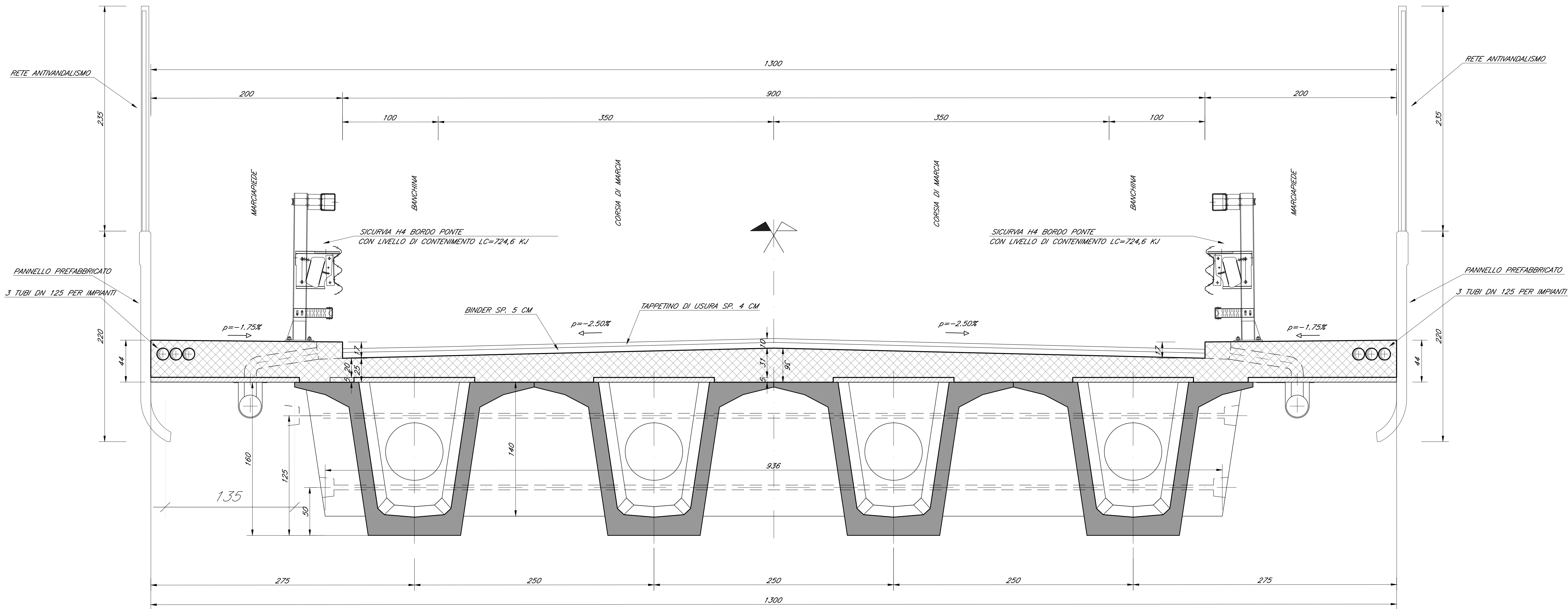
SEZIONE A-A Scala 1:20
