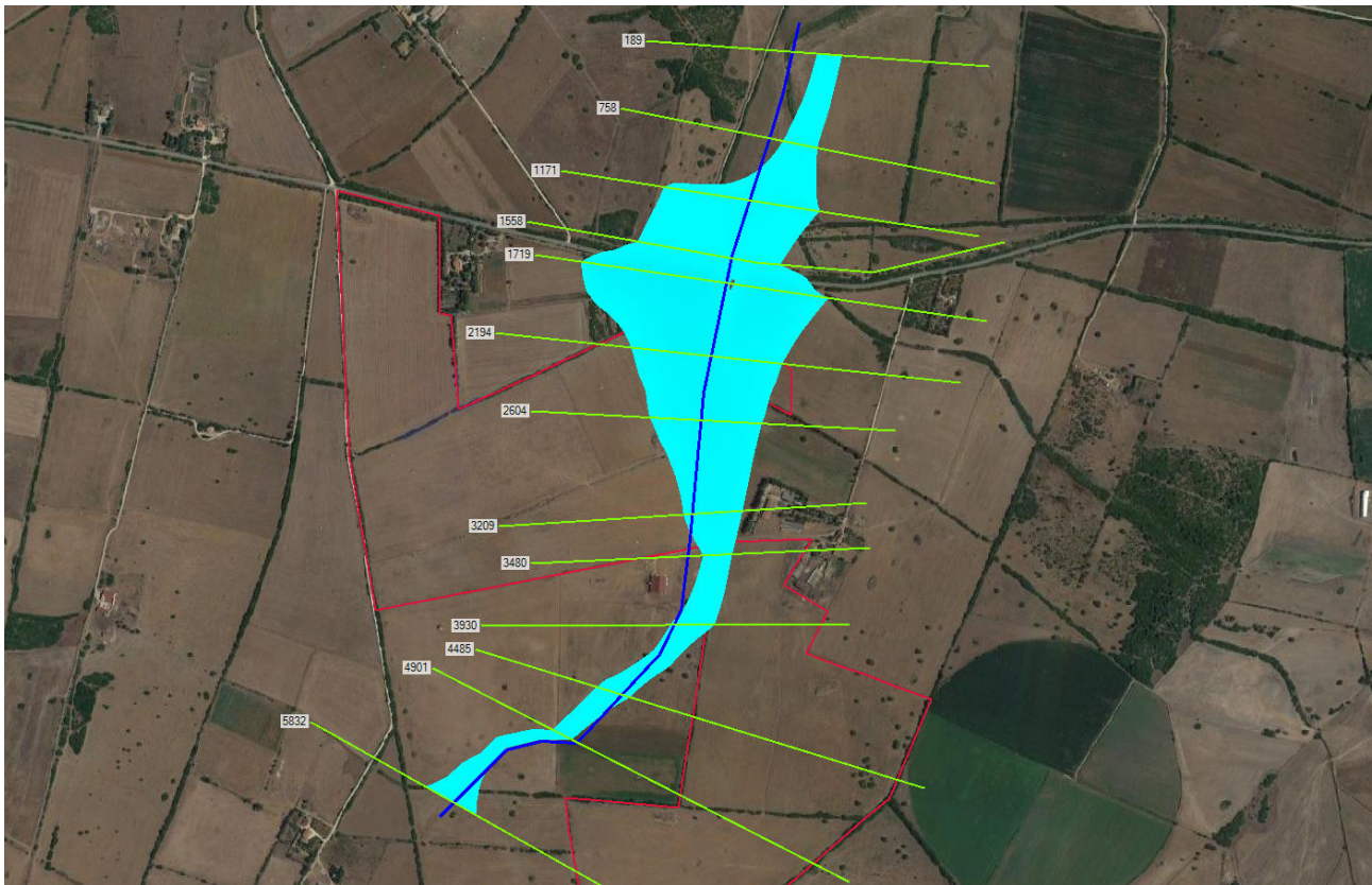
Figura 7 Aree allagate condizione ante-operam, tempo di ritorno 10 anni
