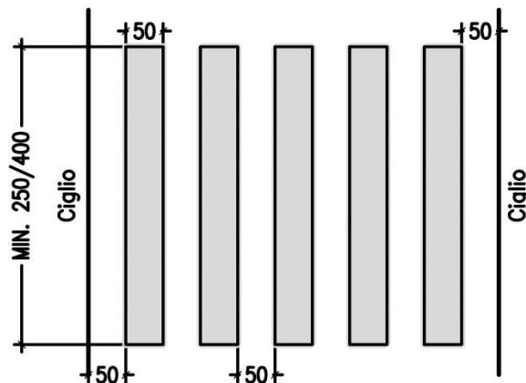
Attraversamenti pedonali Art. 145 (Art. 40 Cod. Str.)
