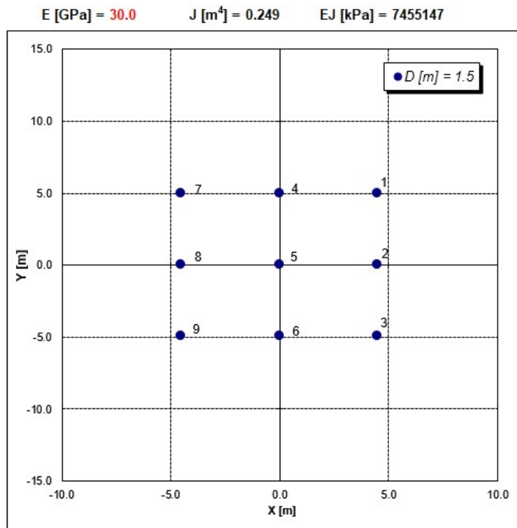
Figura 24 – Fattori di riduzione per effetto gruppo orizzontale
