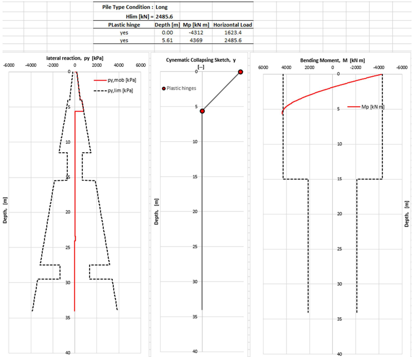
Figura 36 – Verifica carico limite orizzontale – caso 4 – spalla B
