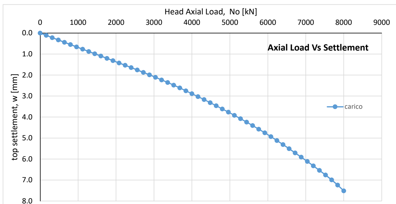
Figura 13 – Curva carico – cedimento palo isolato
