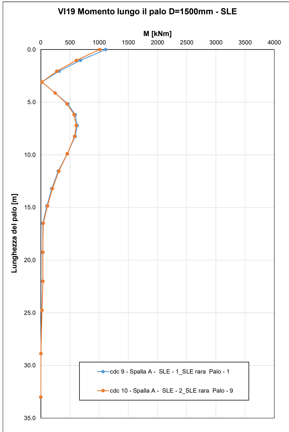
Figura 27 – spalla fissa - Andamento del momento lungo il fusto del palo – SLE
