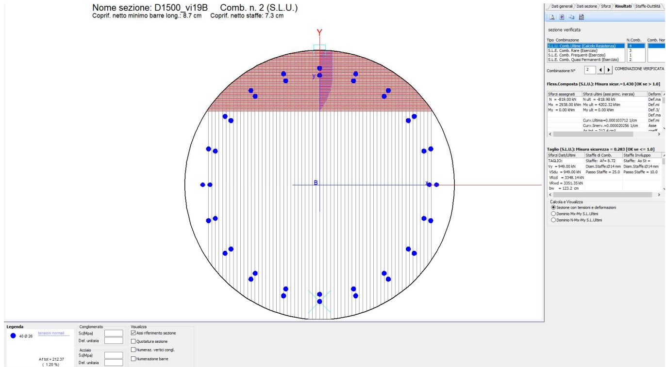
Figura 32 – Verifica strutturale palo spalla mobile
