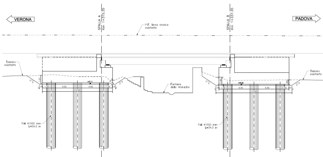
Figura 1 – sezione longitudinale
