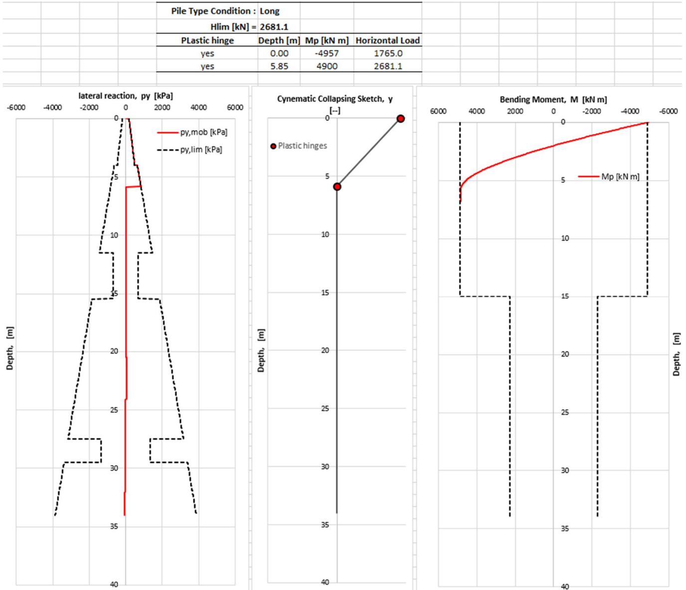
Figura 34 – Verifica carico limite orizzontale – caso 2 – spalla A
