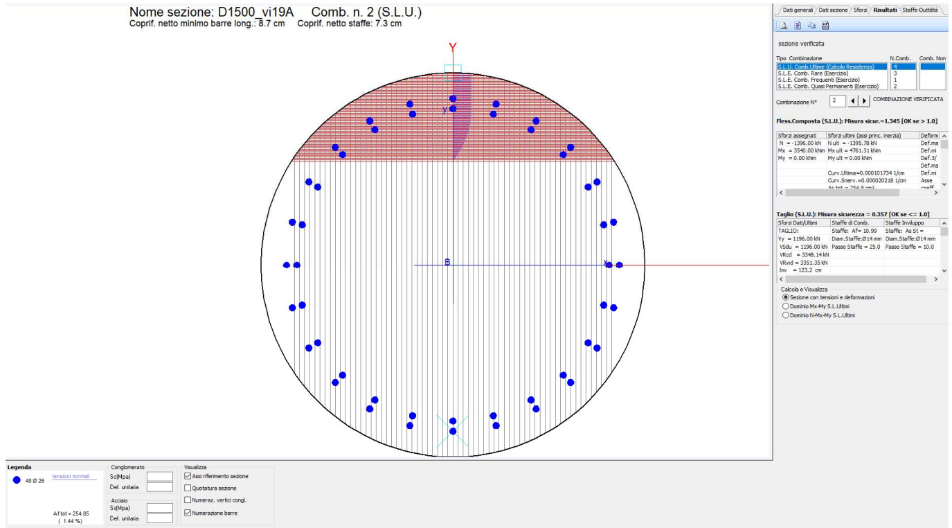
Figura 31 – Verifica strutturale palo spalla fissa
