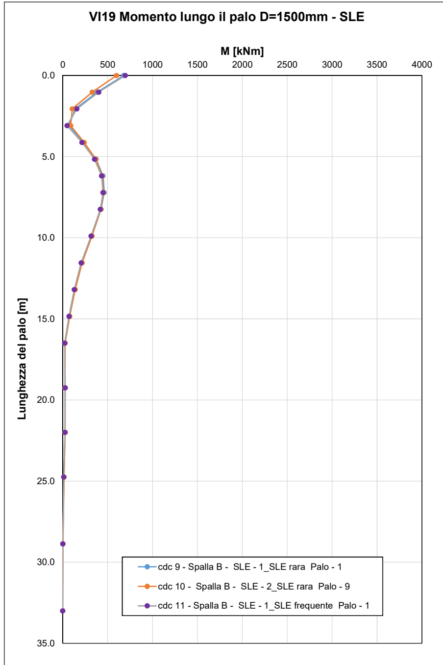
Figura 30 – spalla mobile - Andamento del momento lungo il fusto del palo – SLE
