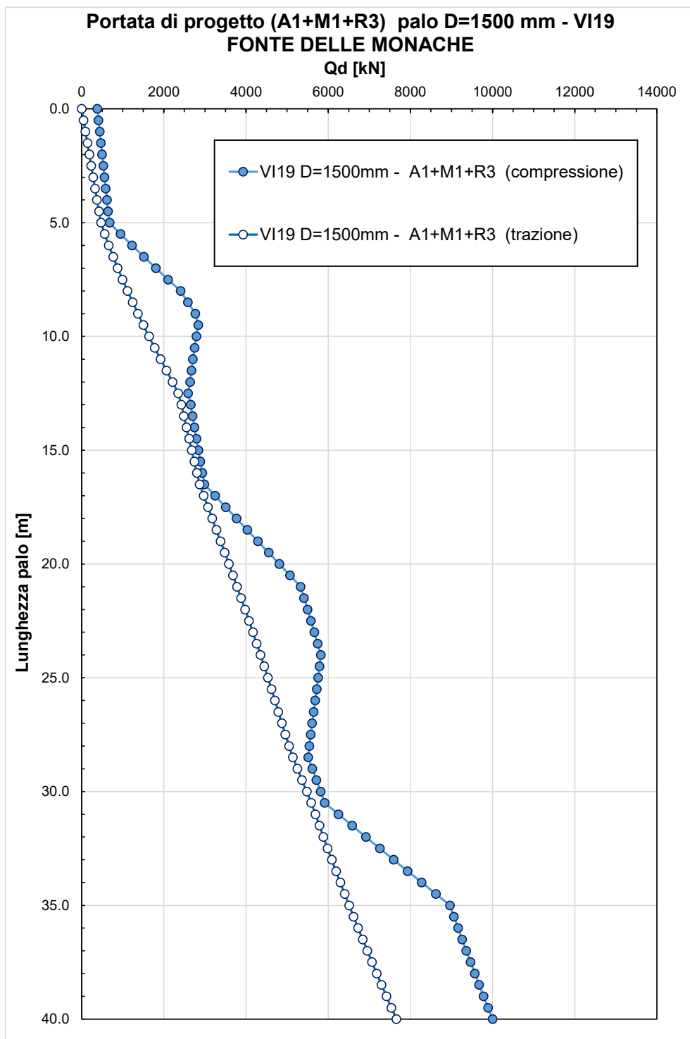
Figura 3 – Portata di progetto palo
