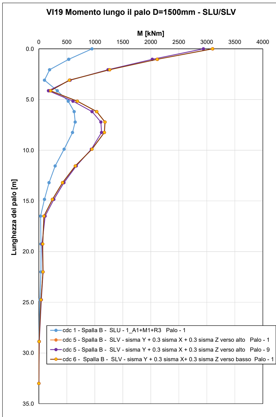
Figura 29 – spalla mobile - Andamento del momento lungo il fusto del palo – SLU/SLV
