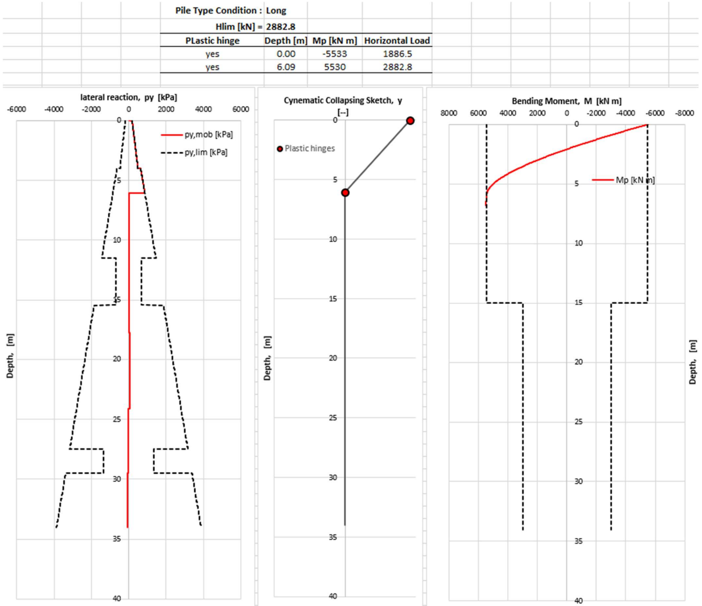
Figura 33 – Verifica carico limite orizzontale – caso 1 – spalla A
