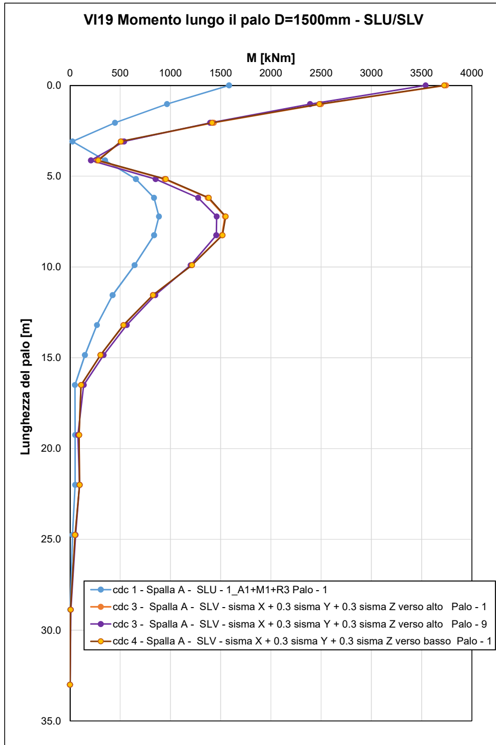
Figura 26 – spalla fissa - Andamento del momento lungo il fusto del palo – SLU/SLV
