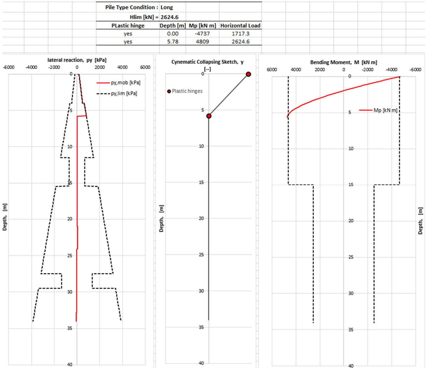
Figura 35 – Verifica carico limite orizzontale – caso 3 – spalla B
