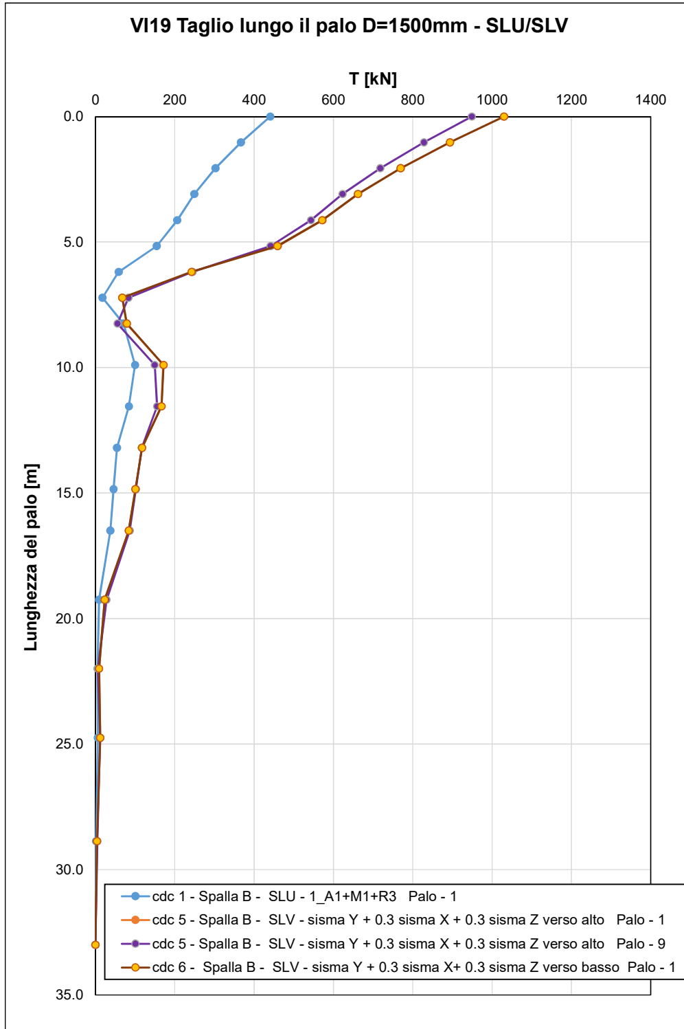
Figura 28 – spalla mobile - Andamento del taglio lungo il fusto del palo – SLU/SLV
