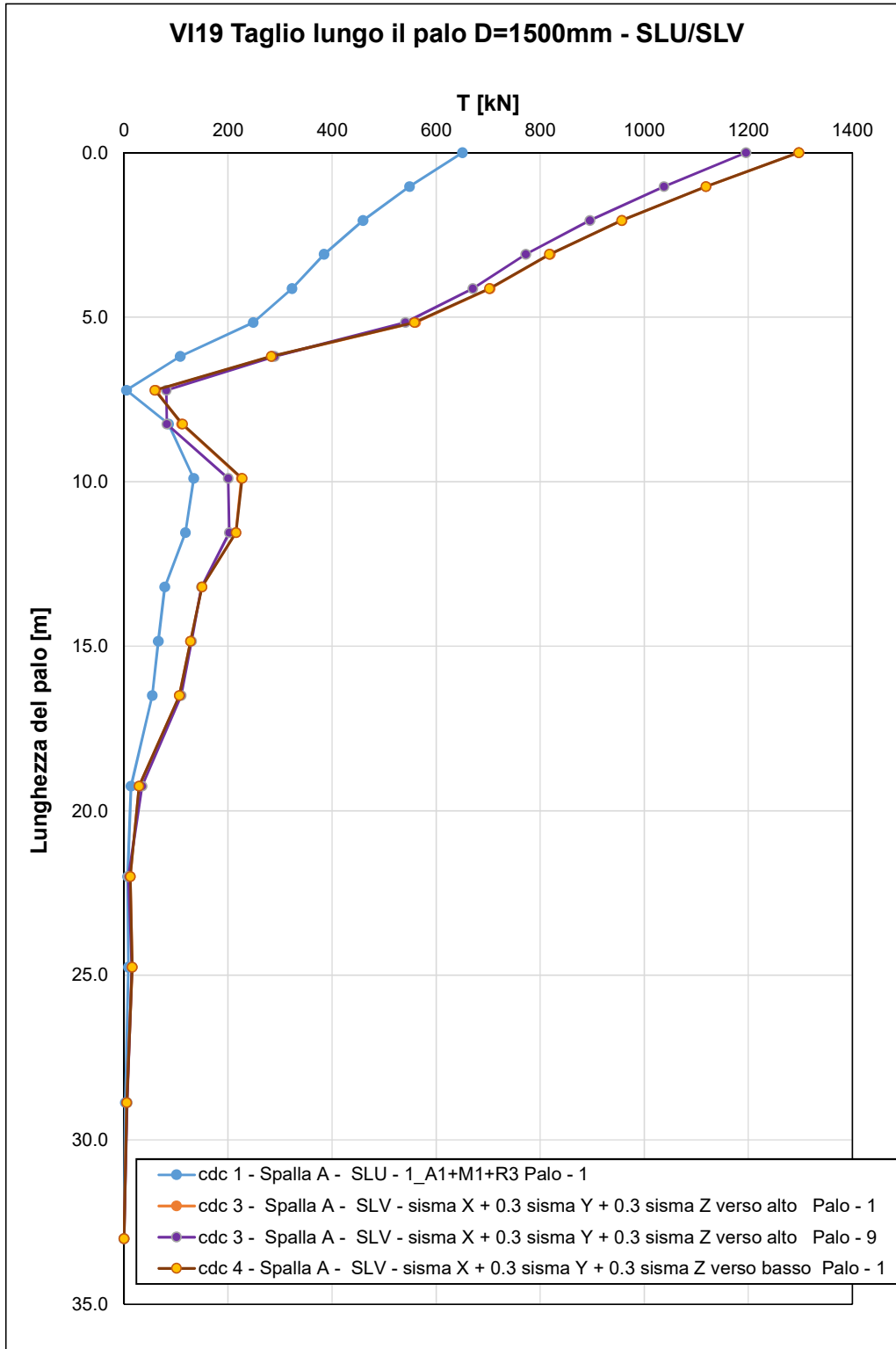
Figura 25 – spalla fissa - Andamento del taglio lungo il fusto del palo – SLU/SLV
