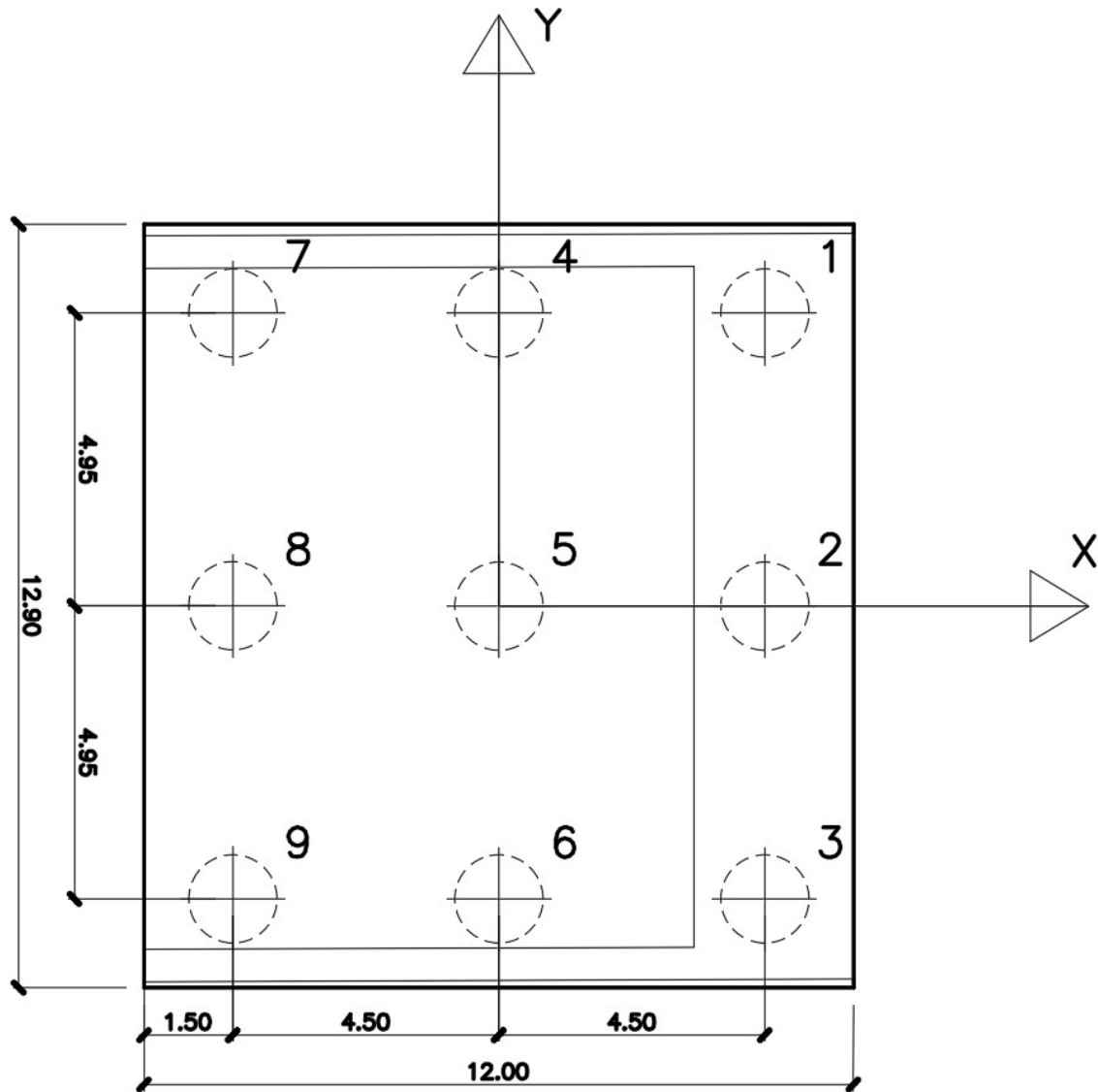
Figura 2 – pianta pali
