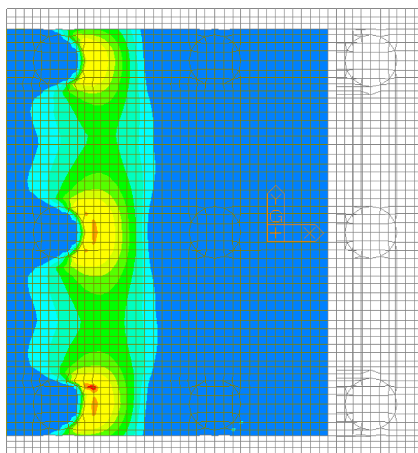
Figura 89 – Involuppo SLE Rara – W-A Moment Bottom Direzione 1
