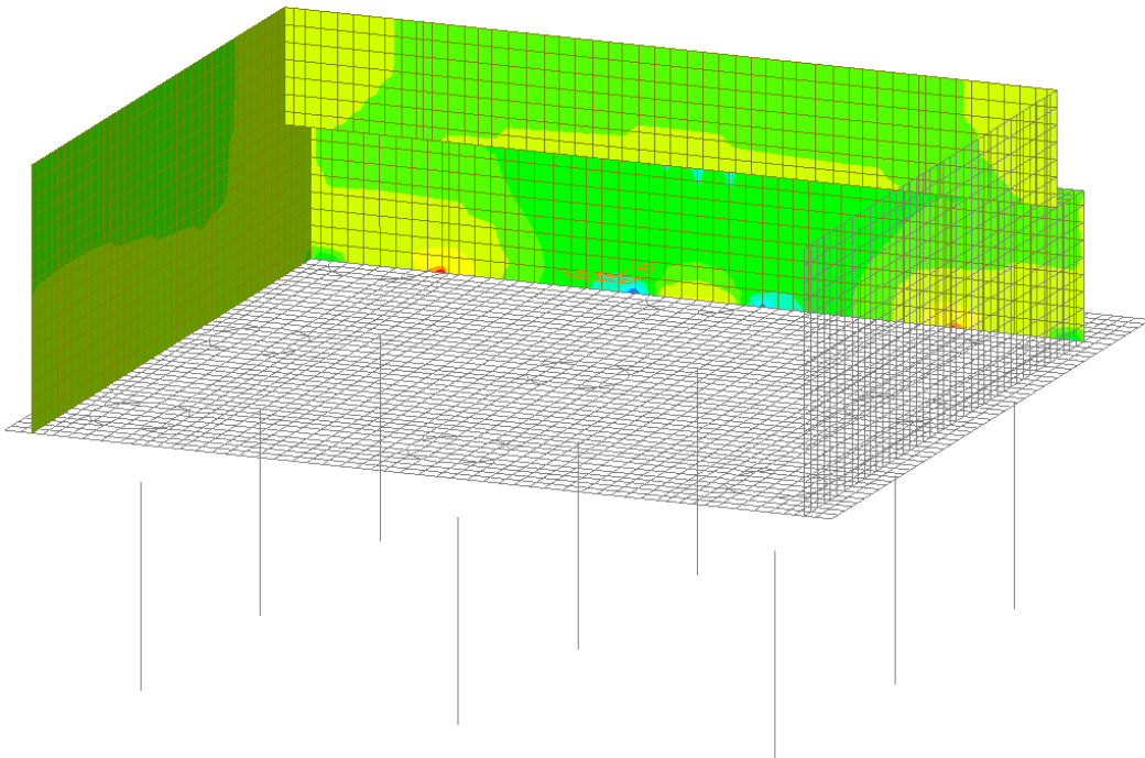
Figura 27 – Involuppo SLU - Mxx
