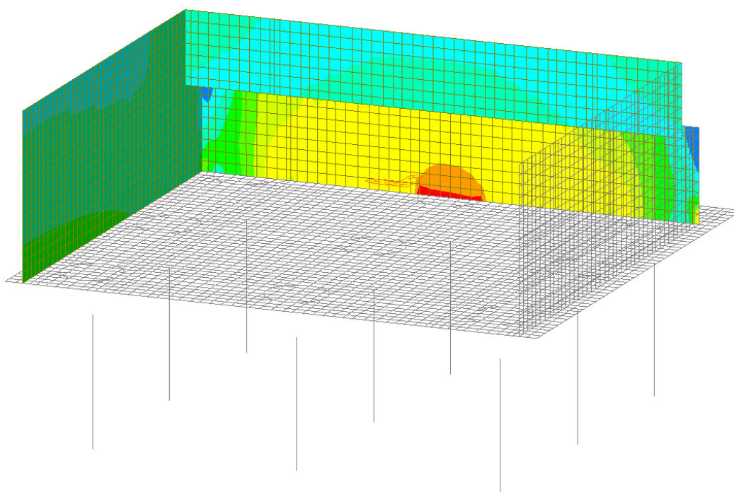
Figura 35 – Involuppo SLE Rara - Myy
