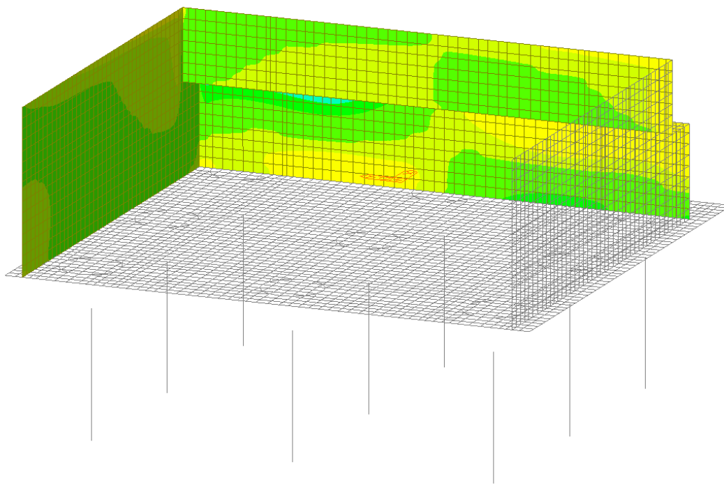
Figura 31 – Involuppo SLU - Vxx
