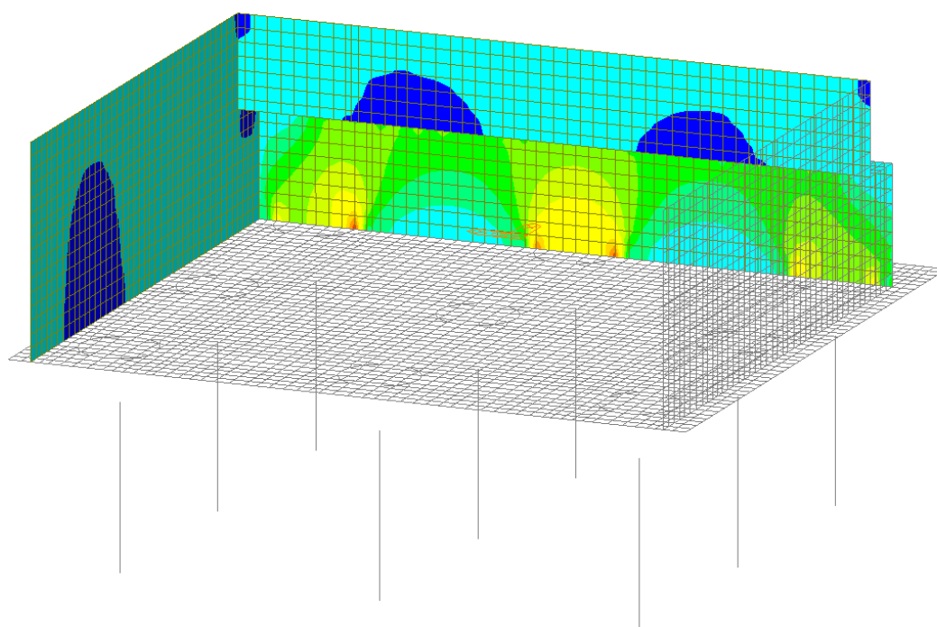
Figura 42 – Involuppo SLE Frequente - Fyy
