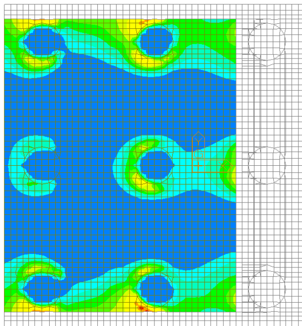
Figura 90 – Involuppo SLE Rara – W-A Moment Top Direzione 2
