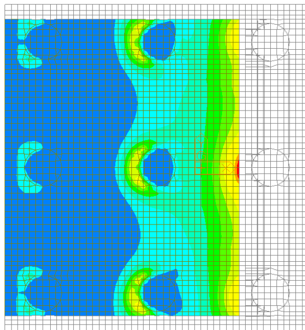
Figura 88 – Involuppo SLE Rara – W-A Moment Top Direzione 1
