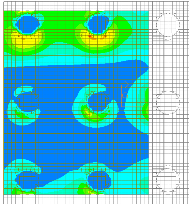
Figura 86 – Inviluppo SLU – W-A Moment Top Direzione 2
