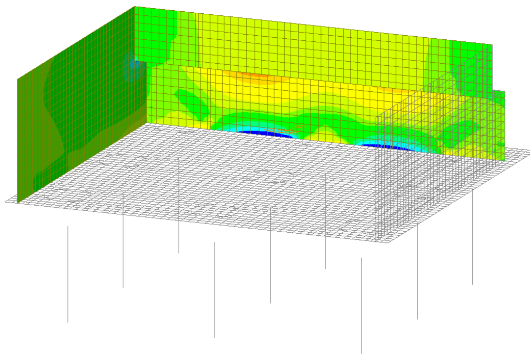
Figura 34 – Involuppo SLE Rara - Fxx
