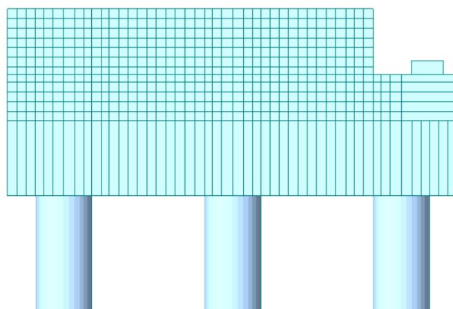
Figura 8 – Vista laterale del modello della spalla
