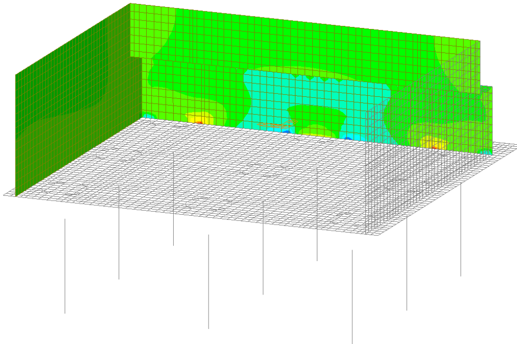
Figura 45 – Involuppo SLE Quasi Permanente - Mxx
