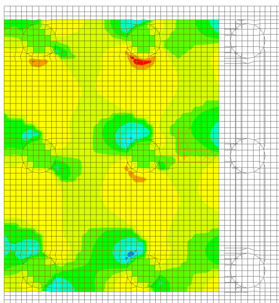
Figura 103 – Involuppo SLU - Vyy
