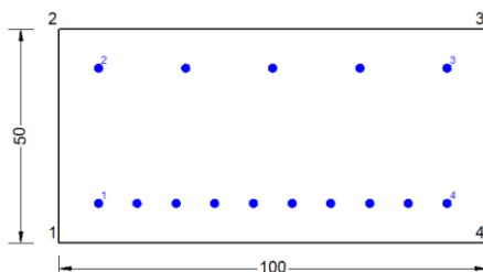
Figura 61 – Sezione implementata in RC-SEC
