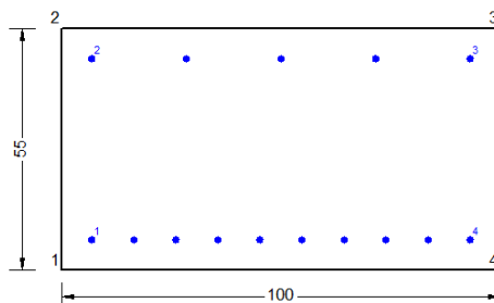
Figura 75 – Sezione implementata in RC-SEC
