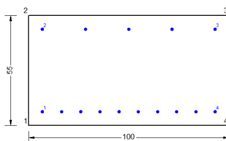
Figura 74 – Sezione implementata in RC-SEC
