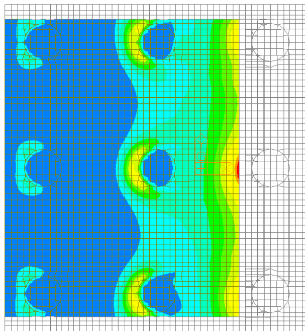
Figura 92 – Involuppo SLE Frequente – W-A Moment Top Direzione 1
