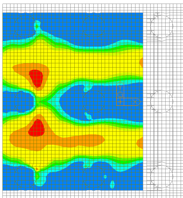
Figura 95 – Involuppo SLE Frequente – W-A Moment Bottom Direzione 2
