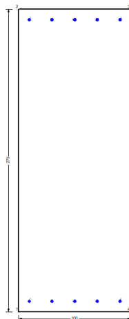
Figura 57 – Sezione implementata in RC-SEC
