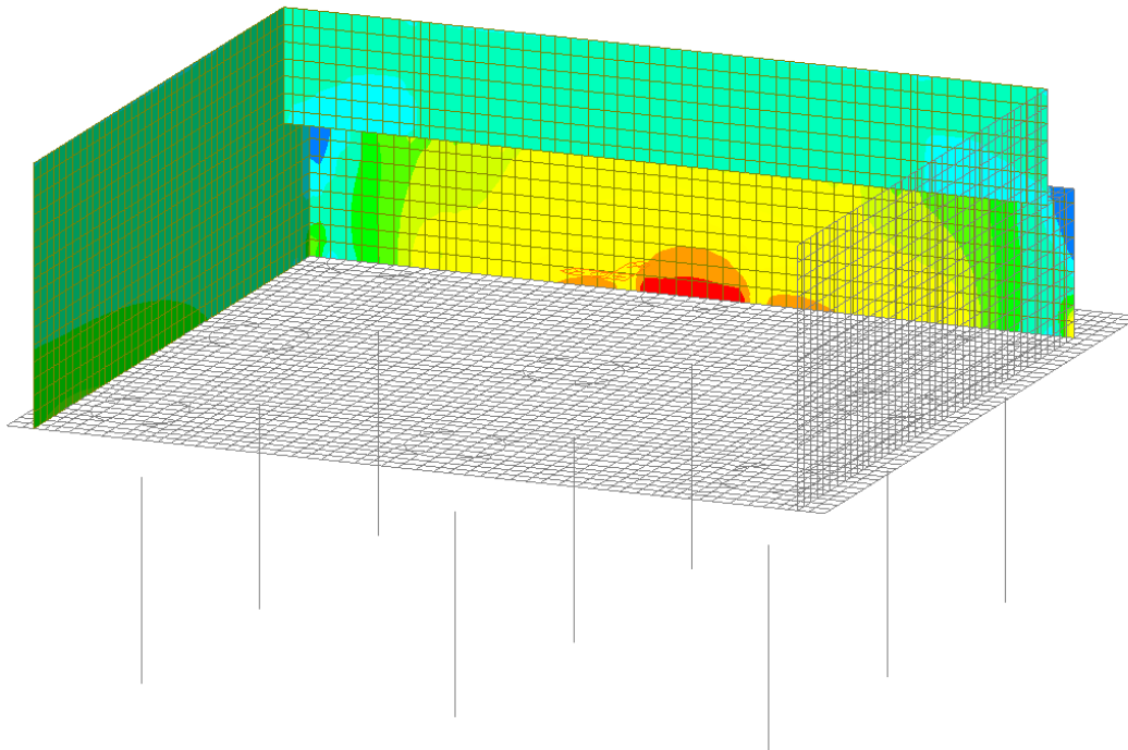
Figura 29 – Involuppo SLU - Myy
