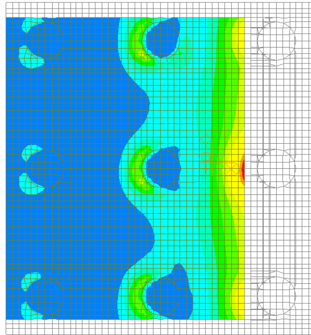
Figura 84 – Inviluppo SLU – W-A Moment Top Direzione 1
