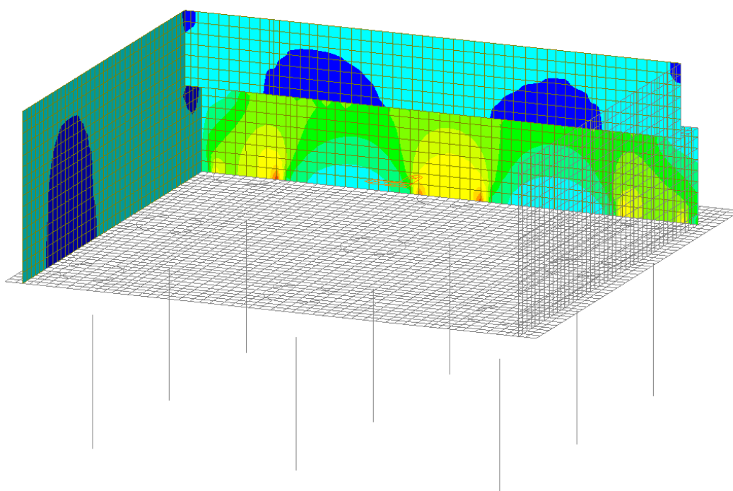
Figura 36 – Involuppo SLE Rara - Fyy
