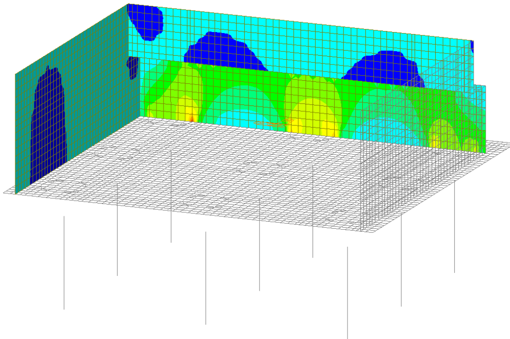
Figura 30 – Involuppo SLU - Fyy
