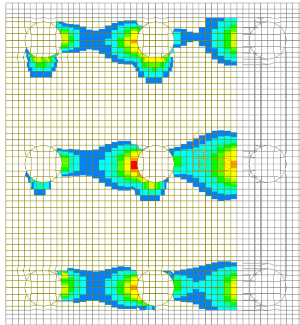
Figura 104 – Involuppo SLU – Vmax maggiore della resistenza a taglio in assenza di armatura trasversale
