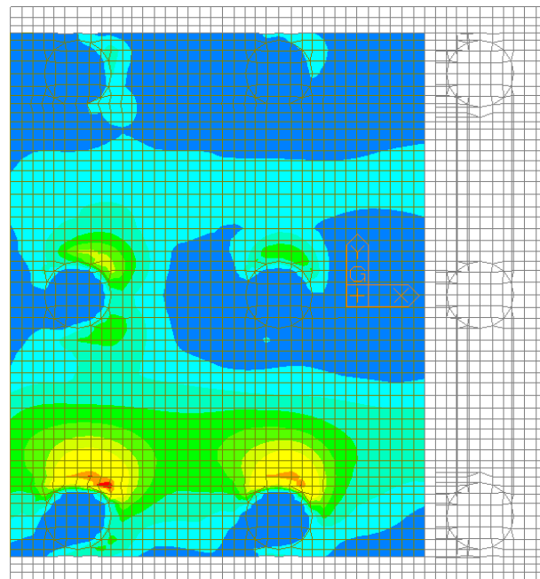
Figura 87 – Inviluppo SLU – W-A Moment Bottom Direzione 2
