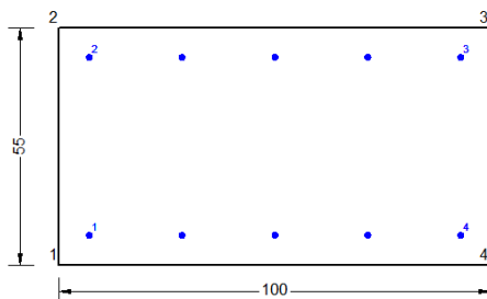
Figura 81 – Sezione implementata in RC-SEC
