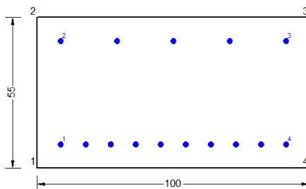
Figura 69 – Sezione implementata in RC-SEC
