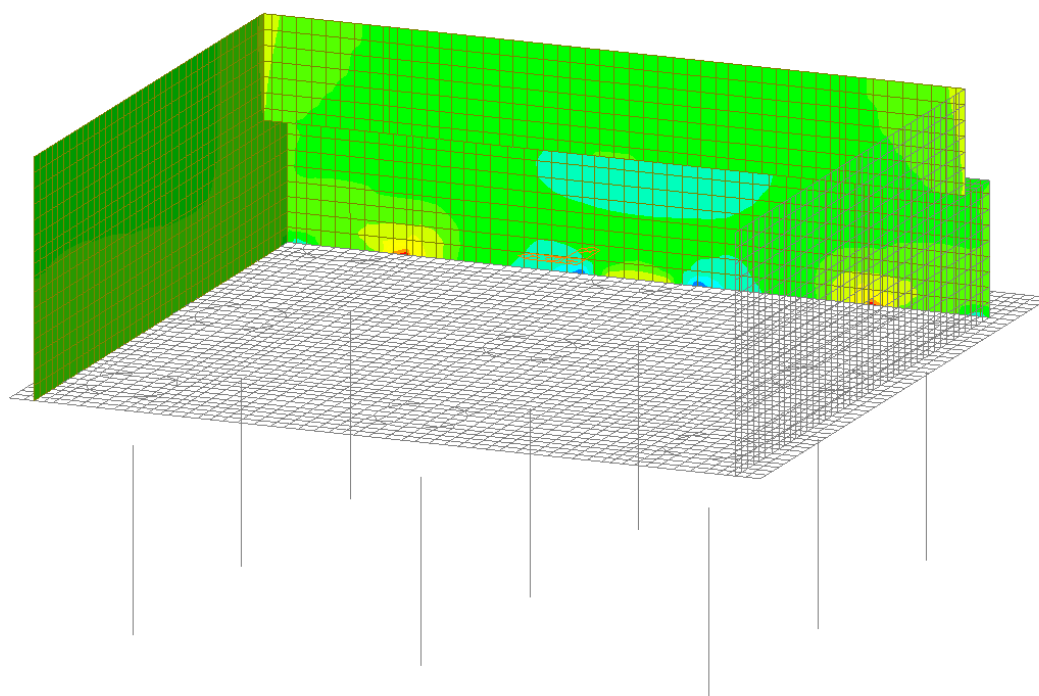
Figura 33 – Involuppo SLE Rara - Mxx
