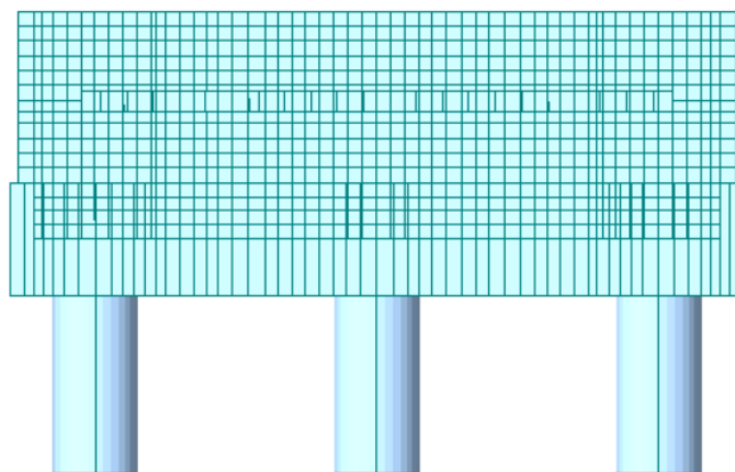
Figura 7 – Vista frontale del modello della spalla
