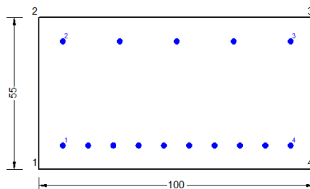
Figura 71 – Sezione implementata in RC-SEC
