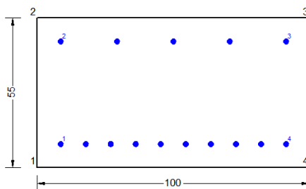
Figura 68 – Sezione implementata in RC-SEC
