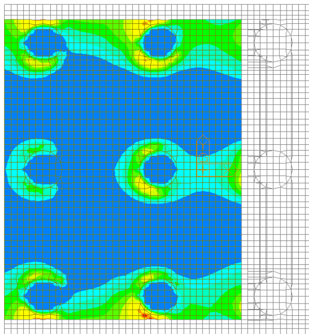
Figura 94 – Involuppo SLE Frequente – W-A Moment Top Direzione 2
