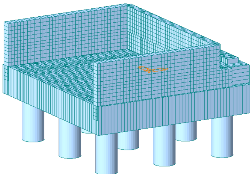
Figura 6 – Vista prospettica del modello della spalla
