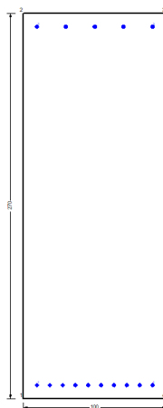
Figura 52 – Sezione implementata in RC-SEC
