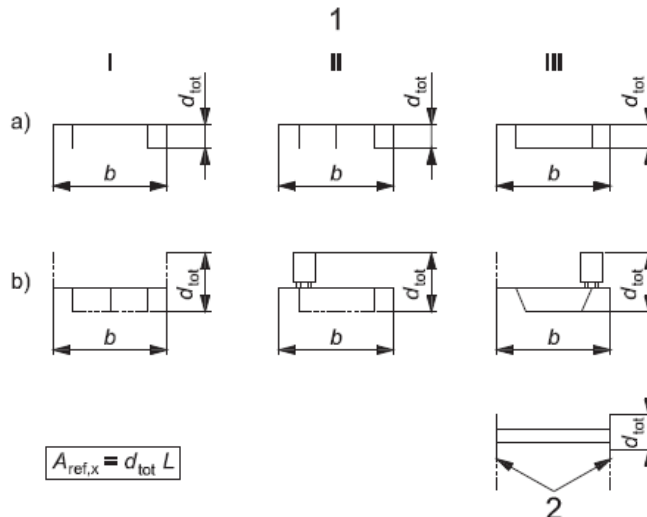
Figura 14 - Area effettiva - Eurocodice 1991-1-4
