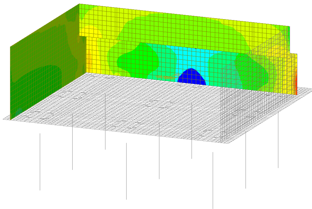
Figura 44 – Involuppo SLE Frequente - V yy
