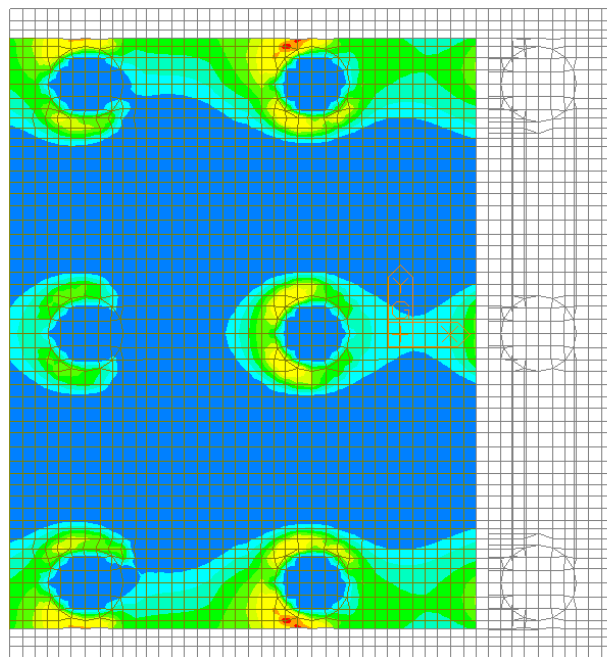
Figura 98 – Involuppo SLE Quasi Permanente – W-A Moment Top Direzione 2
