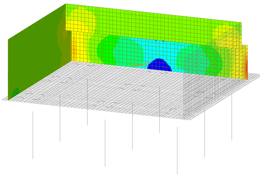
Figura 32 – Involuppo SLU - Vyy
