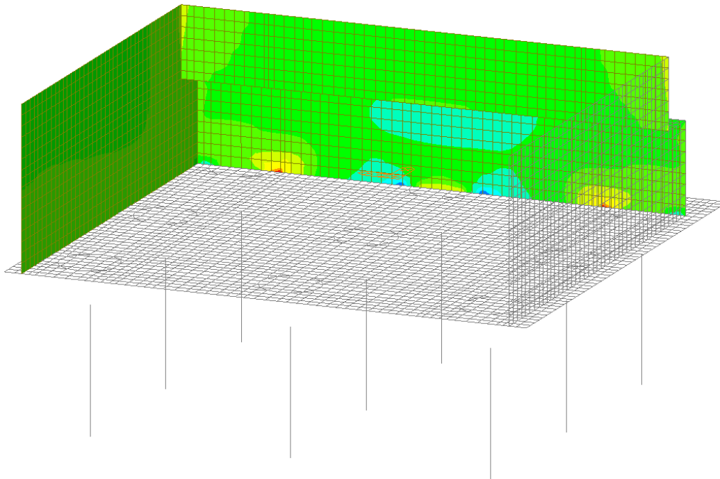
Figura 39 – Involuppo SLE Frequente - Mxx
