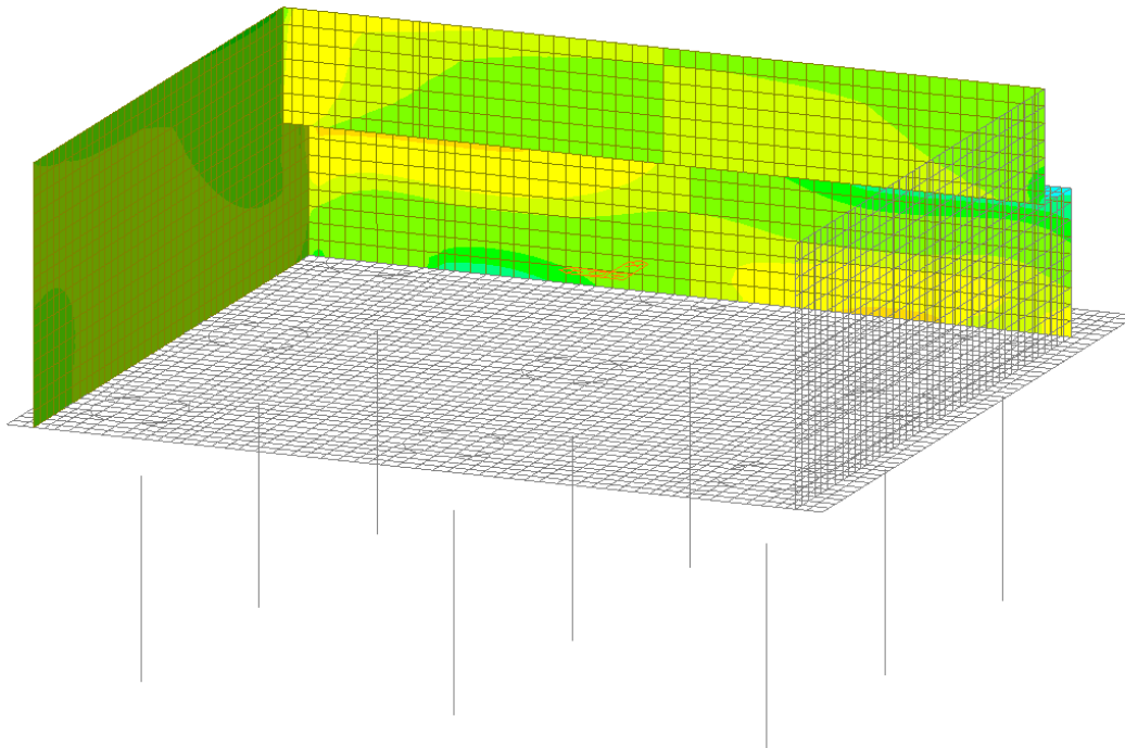
Figura 49 – Involuppo SLE Quasi Permanente - V xx
