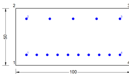
Figura 60 – Sezione implementata in RC-SEC
