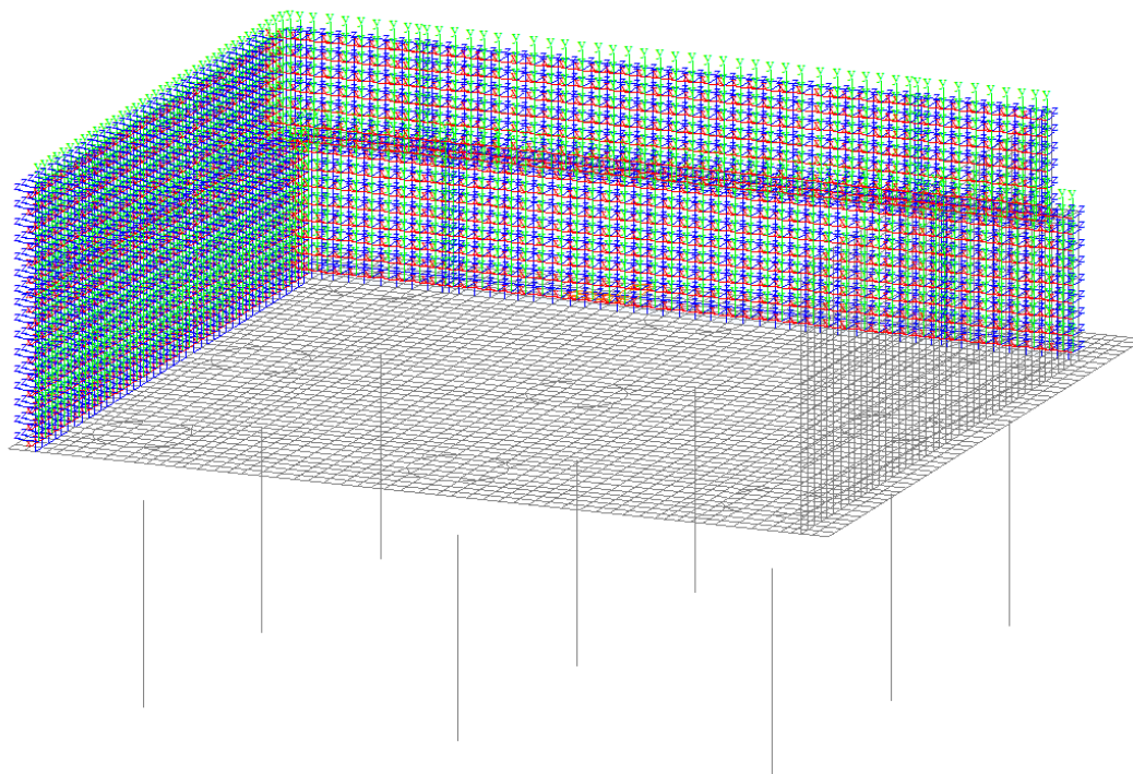
Figura 25 – Assi locali per gli elementi dei muri
