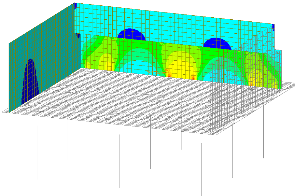
Figura 48 – Involuppo SLE Quasi Permanente - Fyy
