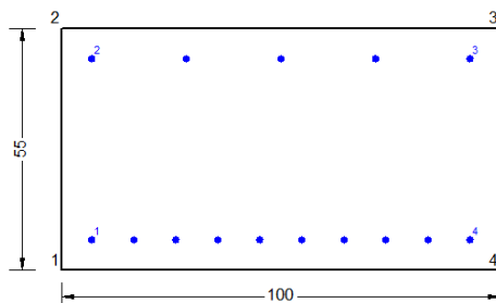
Figura 79 – Sezione implementata in RC-SEC
