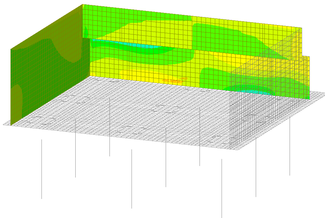
Figura 43 – Involuppo SLE Frequente - V xx
