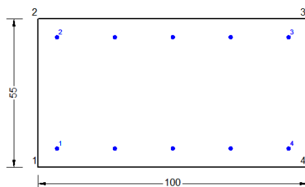
Figura 83 – Sezione implementata in RC-SEC
