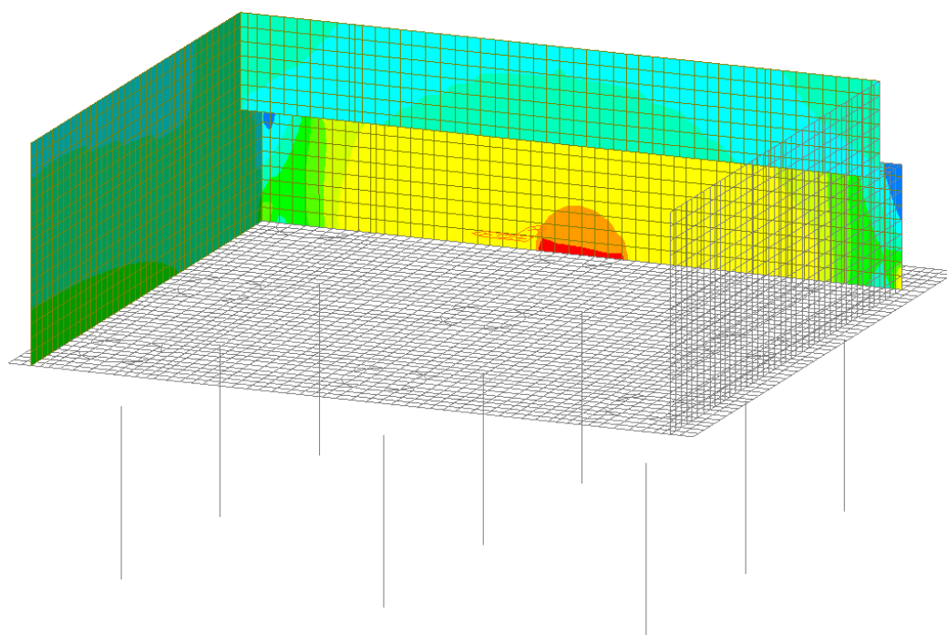
Figura 41 – Involuppo SLE Frequente - Myy
