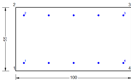
Figura 82 – Sezione implementata in RC-SEC
