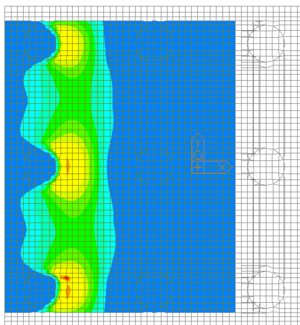
Figura 93 – Involuppo SLE Frequente – W-A Moment Bottom Direzione 1
