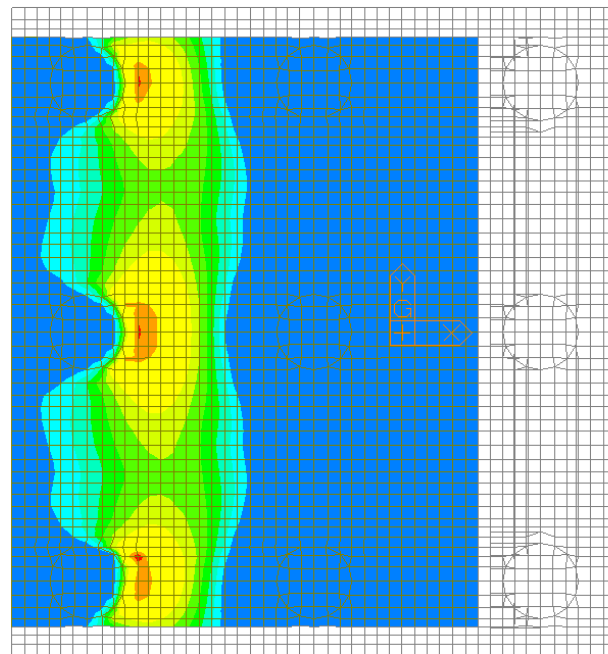
Figura 97 – Inviluppo SLE Quasi Permanente – W-A Moment Bottom Direzione 1
