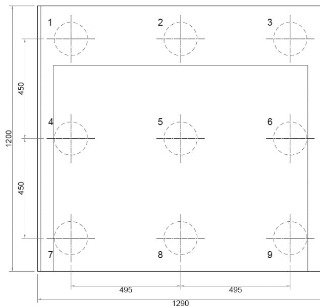
Figura 106 – Disposizione e numerazione dei pali di fondazione
