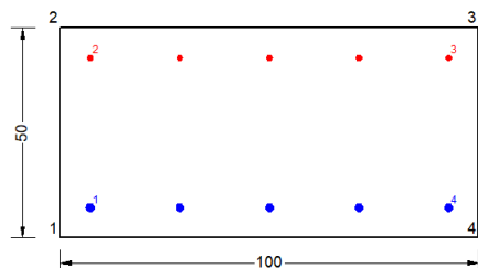
Figura 66 – Sezione implementata in RC-SEC
