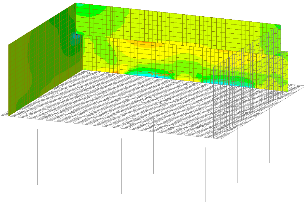
Figura 28 – Involuppo SLU - Fxx
