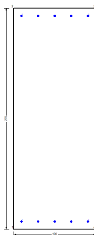
Figura 56 – Sezione implementata in RC-SEC
