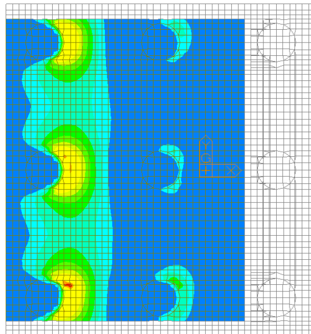
Figura 85 – Inviluppo SLU – W-A Moment Bottom Direzione 1
