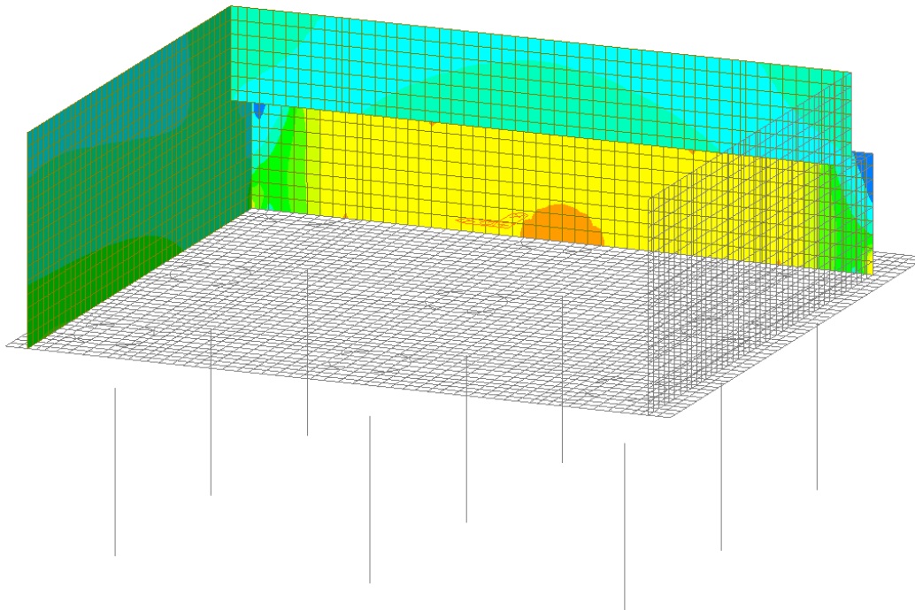
Figura 47 – Involuppo SLE Quasi Permanente - Myy
