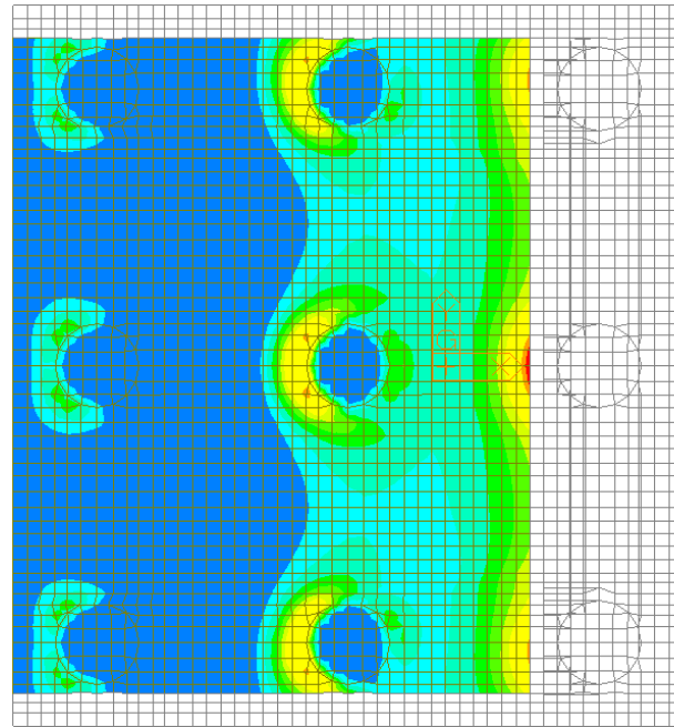
Figura 96 – Inviluppo SLE Quasi Permanente – W-A Moment Top Direzione 1
