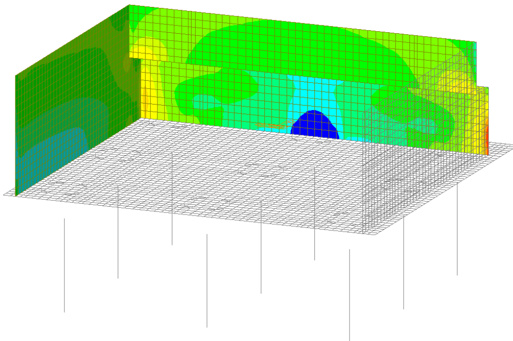
Figura 50 – Involuppo SLE Quasi Permanente - V yy
