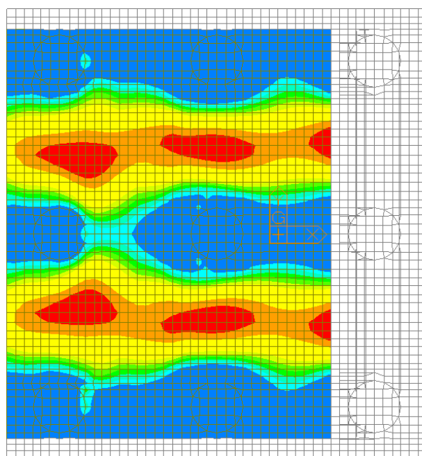
Figura 99 – Involuppo SLE Quasi Permanente – W-A Moment Bottom Direzione 2
