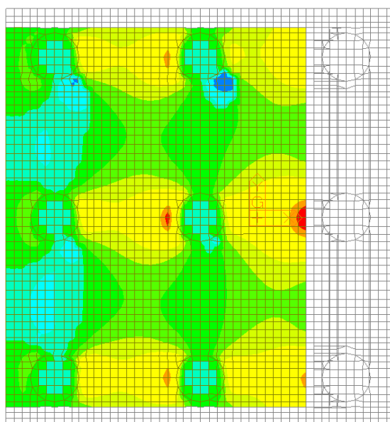
Figura 102 – Involuppo SLU - Vxx
