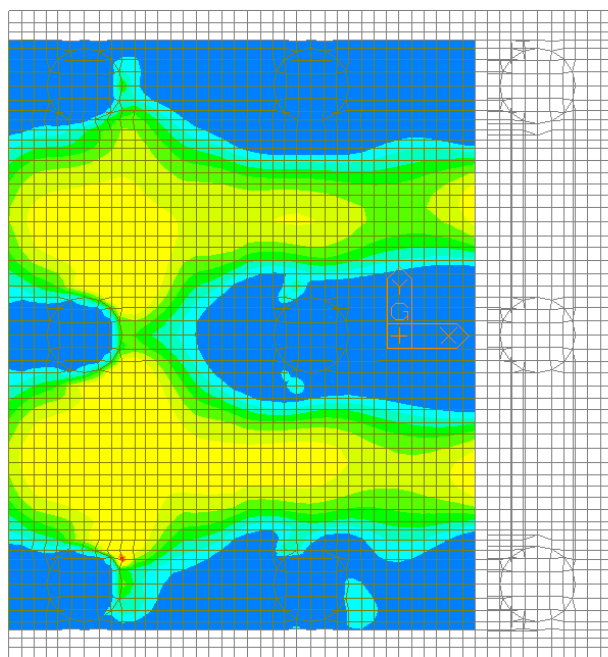
Figura 91 – Involuppo SLE Rara – W-A Moment Bottom Direzione 2
