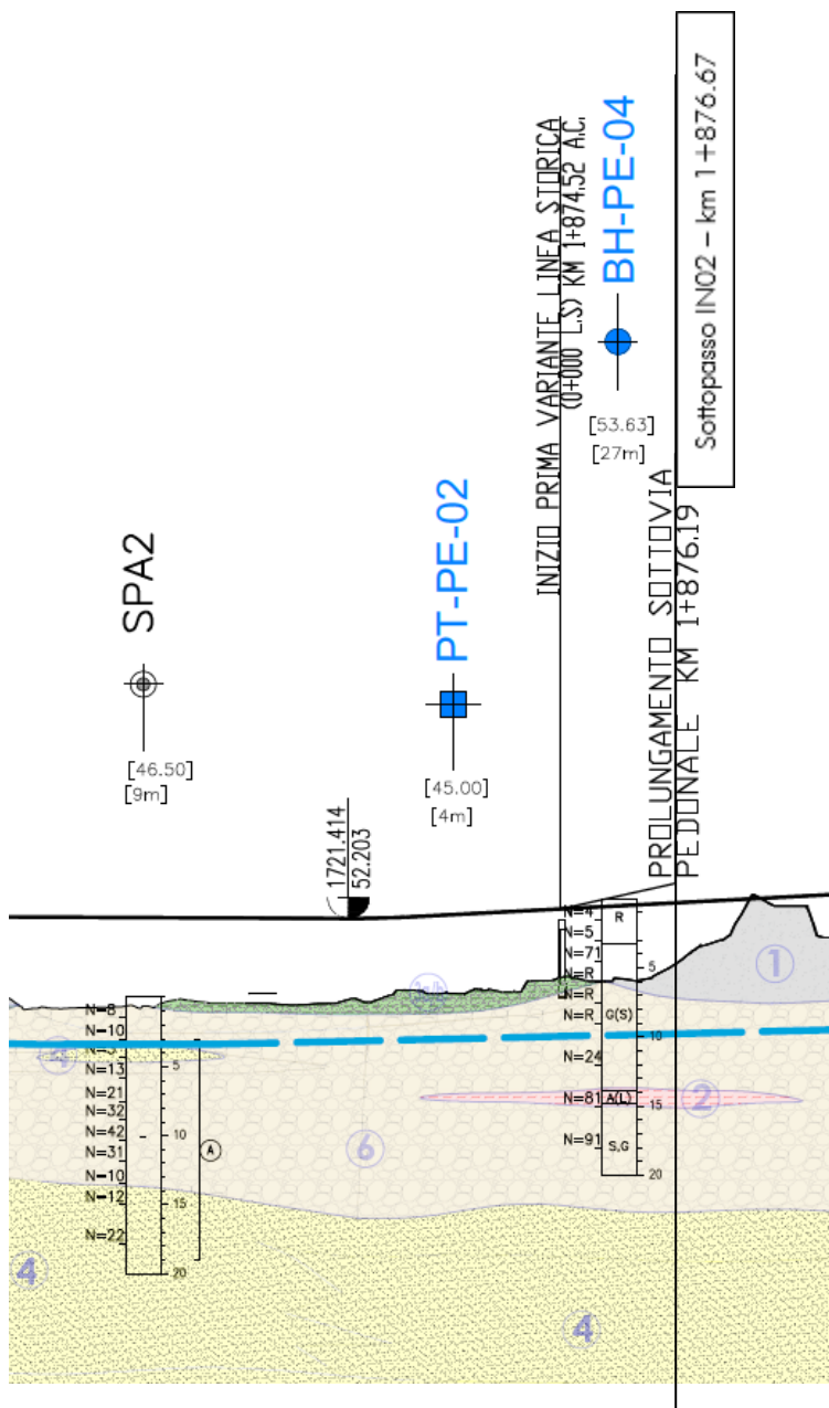
Figura 10: Profilo stratigrafico del tracciato in corrispondenza della progressiva dell'opera in esame
