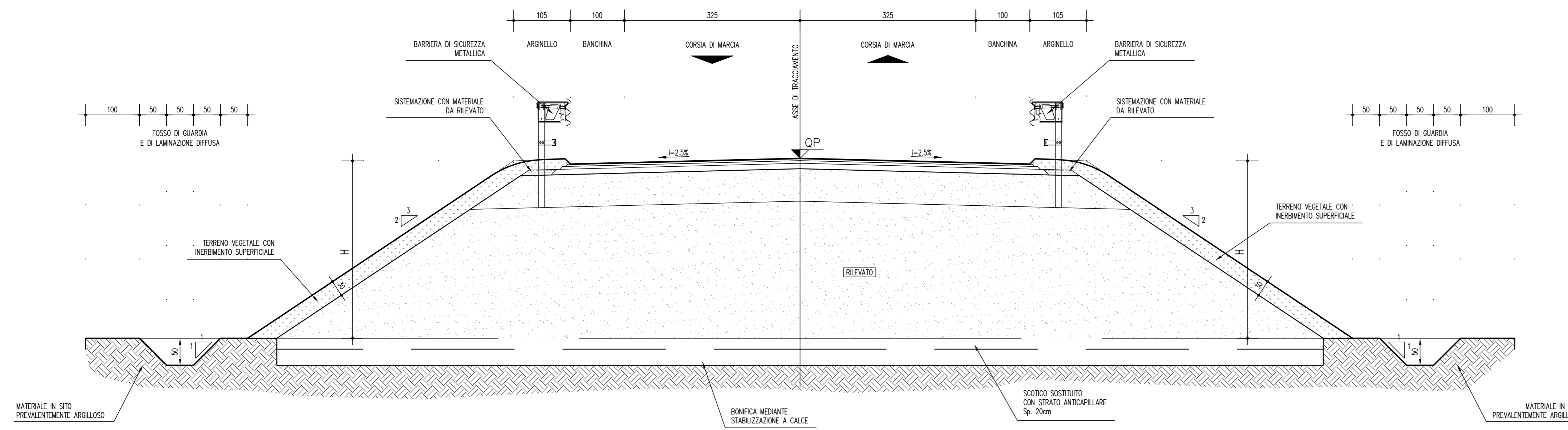
SEZIONE TIPO IN RETTIFILLO CON RILEVATO 1.00m < H < 7.00m scala 1:50
