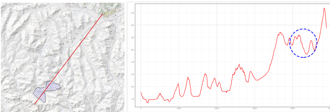
Figura 61 – sezione trasversale (non in scala) dal recettore 3 all'impianto di progetto (blu – area impianto)
