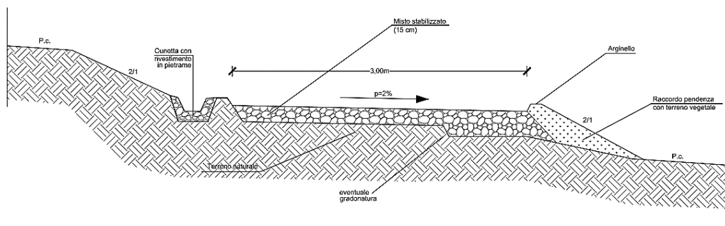
Figura 34 - Sezione tipo strade interne al sito, tipologia a mezza costa (Fonte: ns elaborazione)
