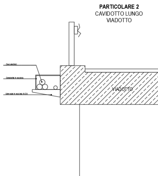
Figura 38 - Particolari risoluzione interferenze
