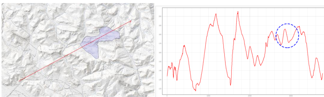
Figura 67 – sezione trasversale (non in scala) dal recettore 5 all'impianto di progetto (blu – area impianto)
