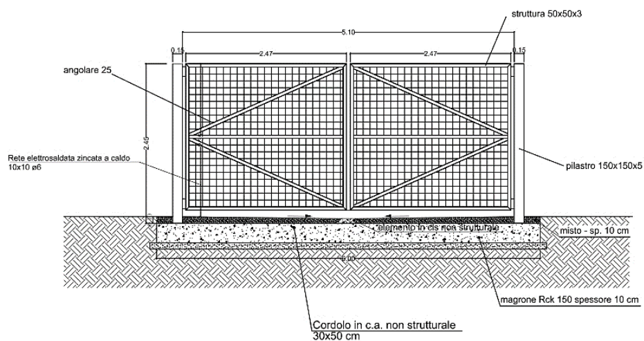
Figura 32 - Cancelli di cantiere. (Fonte: ns elaborazione)
