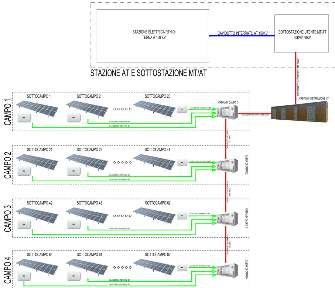
Figura 36 - Schema delle connessioni elettriche
