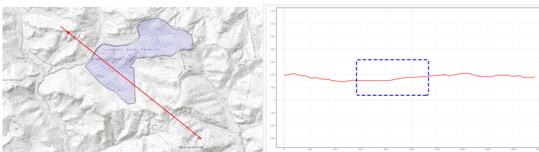
Figura 68 - sezione longitudinale (in scala) all'impianto di progetto (blu – area impianto)
