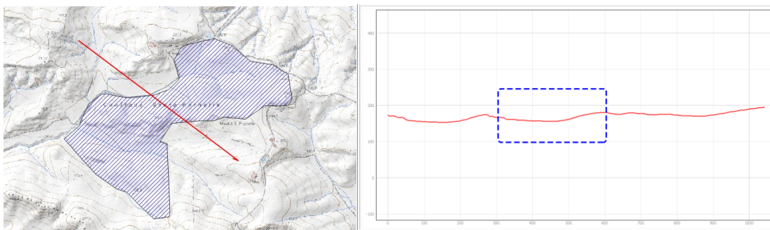
Figura 64 – sezione trasversale (non in scala) dal recettore 4 all'impianto di progetto (blu – area impianto)
