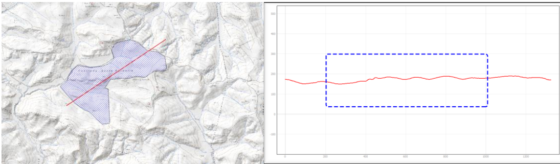
Figura 59 - sezione longitudinale (in scala) all'impianto di progetto (blu – area impianto)
