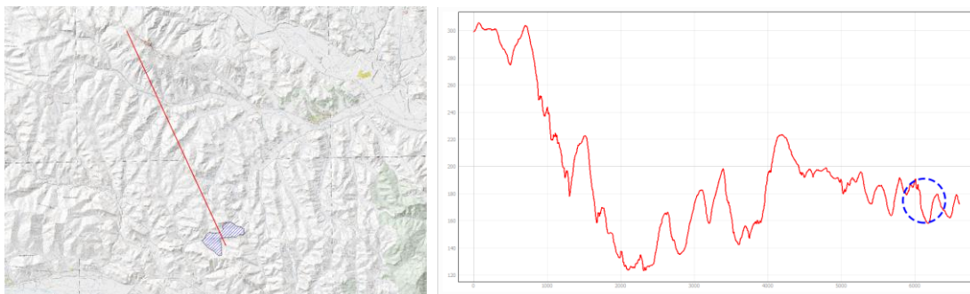
Figura 58 – sezione trasversale (non in scala) dal recettore 2 all'impianto di progetto (blu – area impianto)
