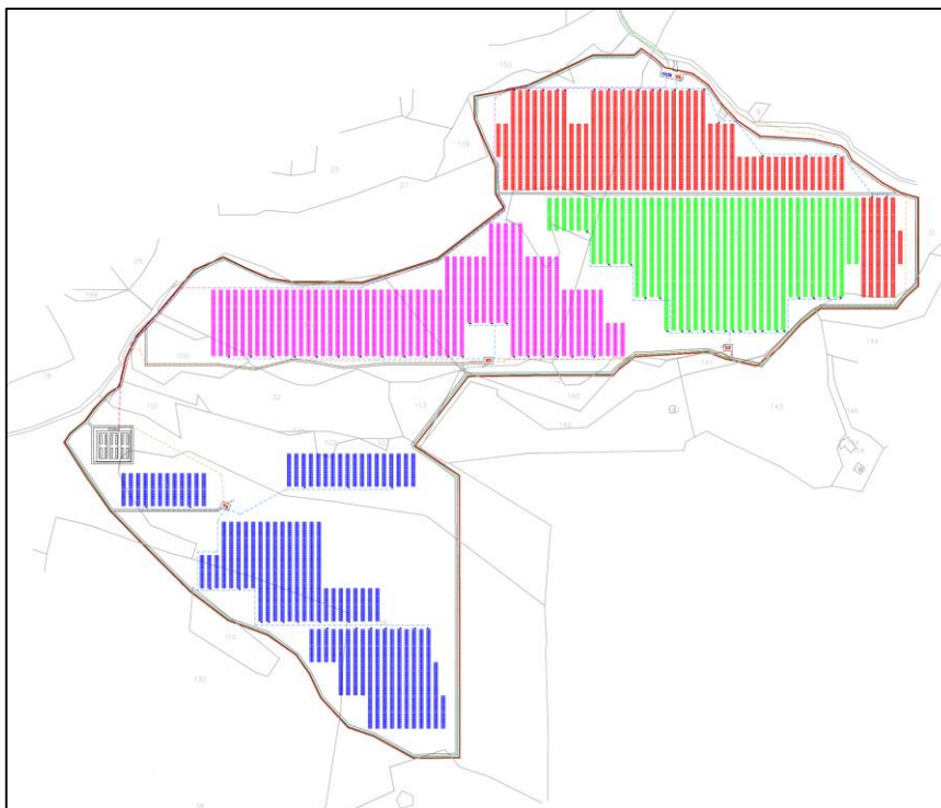
Figura 1 - Planimetria impianto agrivoltaico
