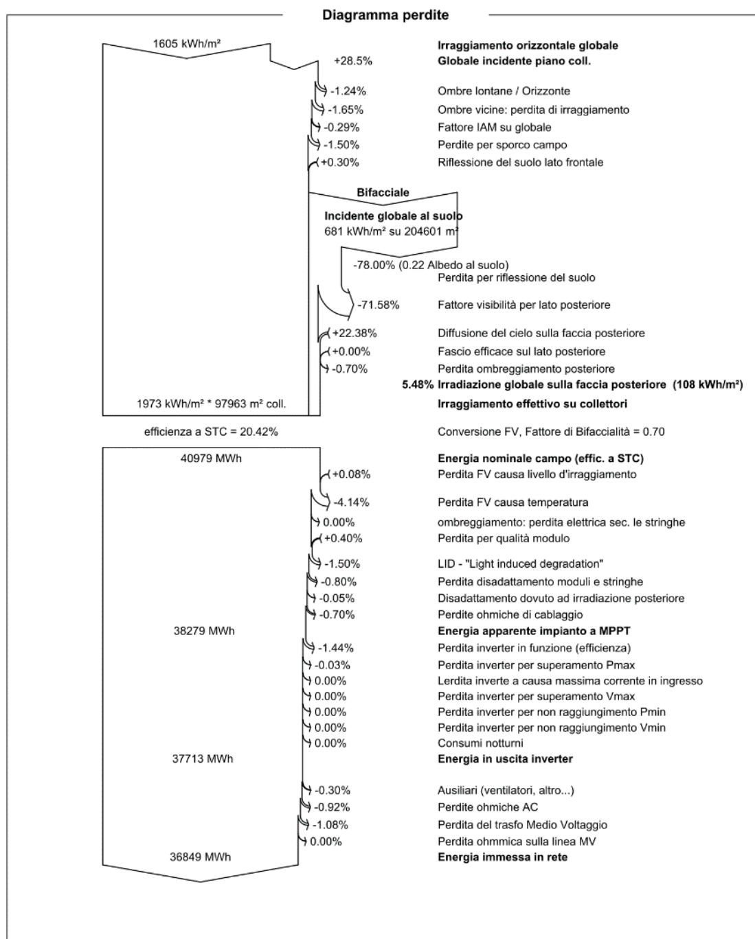
Figura 2- Calcoli PVSyst
