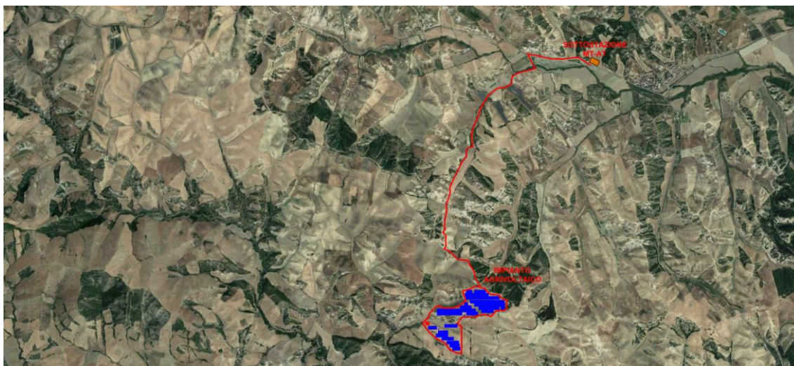
Figura 1 - Inquadramento su ortofoto dell'impianto (stralcio tavola A12a1-3)
